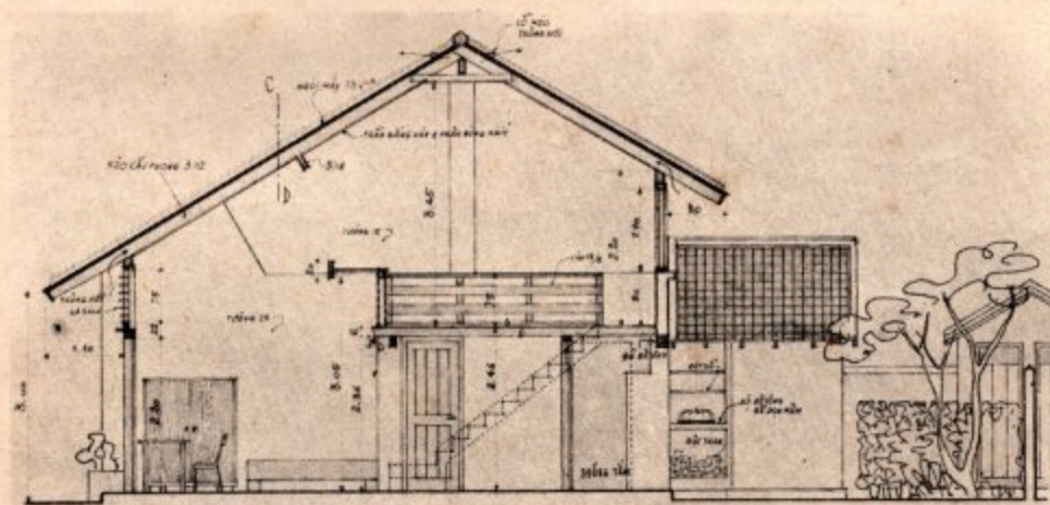
THIẾT ĐỒ DỌC THEO AB
