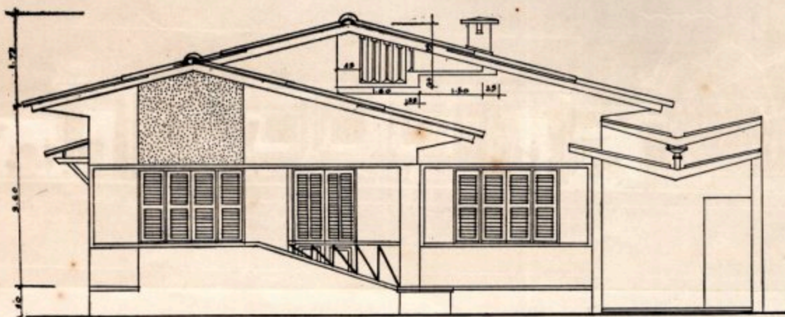
CHÍNH DIỆN
