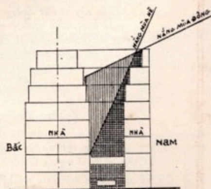
HÌNH SỐ "4"
