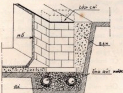
HÌNH SỐ "1"
