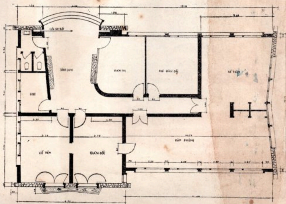
BÌNH ĐỒ
