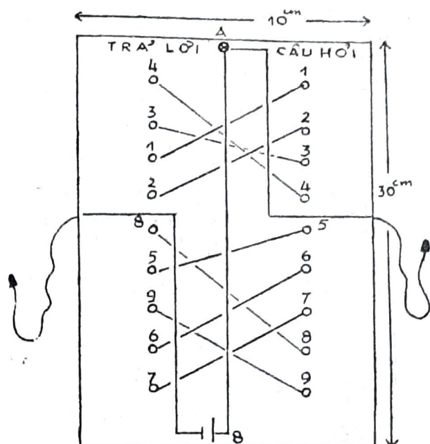
Sơ đồ phía sau máy kiểm tra trí nhớ
