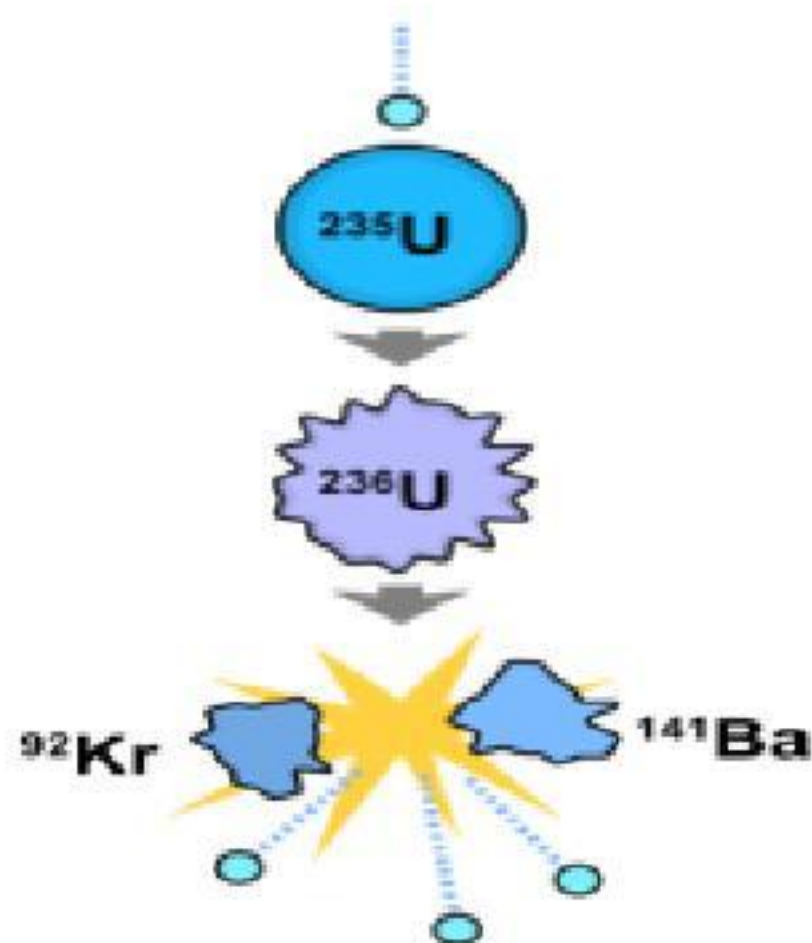
Hình 1 : Sơ đồ phản ứng nguyên tử
