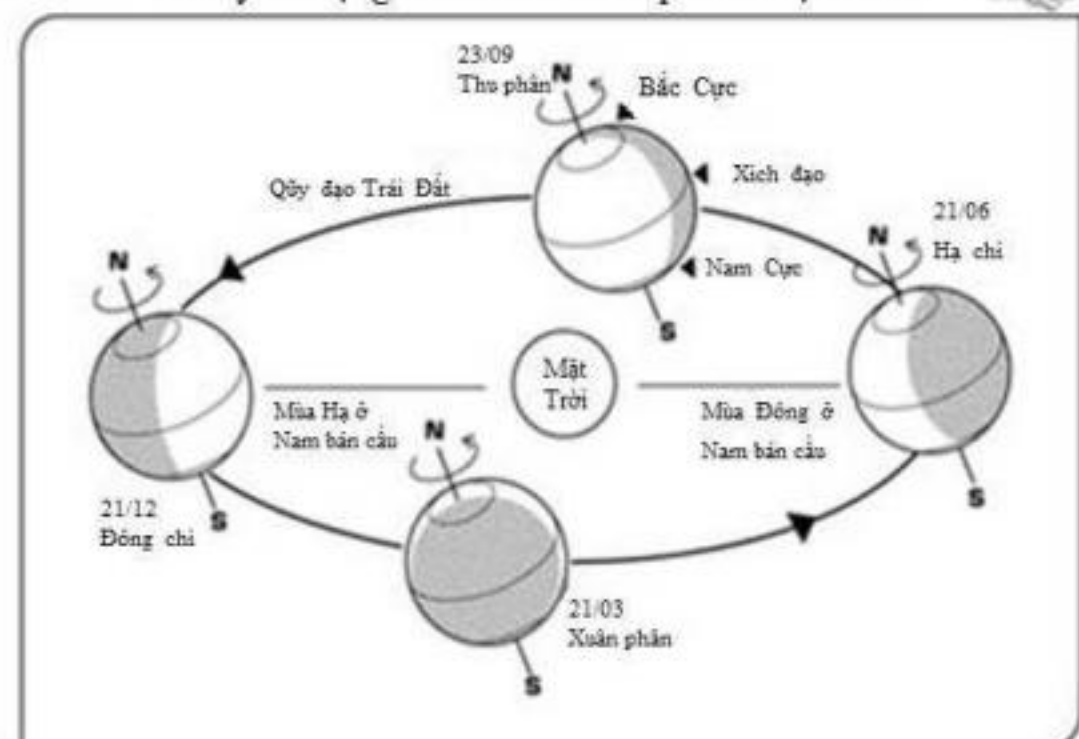
Chuyển động của Trái Đất quanh Mặt Trời
