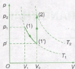
Hình 31.3. Đồ thị biểu diễn quá trình biến đổi trạng thái trên Hình 31.2 trong hệ tọa độ (p, V) .
