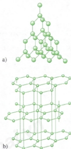
Hình 34.3 Cấu trúc tinh thể
