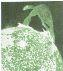
Hình 28.8. Trạng thái plasma trên Mặt Trời.
