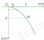
Hình 15.2. Quỹ đạo parabol của vật ném ngang.
