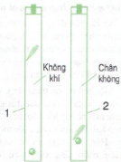
Hình 4.1. Ống Niu-tơn
