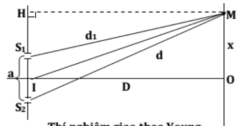
Thí nghiệm giao thoa Young
