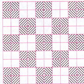
Hình 2. Tô màu 2 \times 2 cho bàn cờ 10 \times 10
