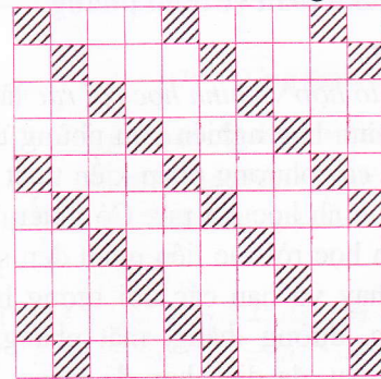
Hình 3. Một cách tô màu cho bàn cờ 10 \times 10
