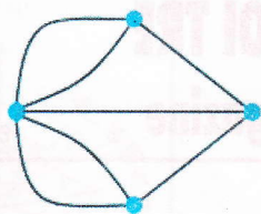
Mô hình về bài toán bảy chiếc cầu ở Königsberg
