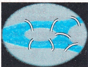
Mô hình về bài toán bảy chiếc cầu ở Königsberg
