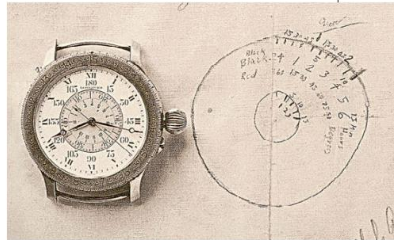
Bảng phác thảo đồng hồ Hour Angle Watch của Charles Lindbergh
