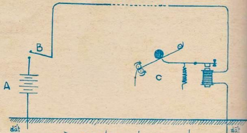
SƠ ĐỒ HỆ THỐNG MÁY ĐIỆN BÁO
