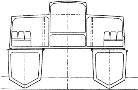
Hình 2.29 Mặt cắt ngang tàu hai thân
