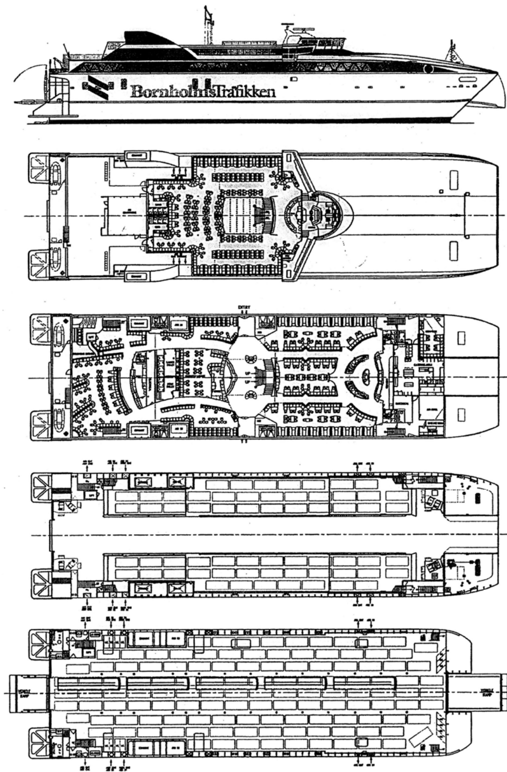
Hình 2.8 Bố trí chung “Villum Clausen”
