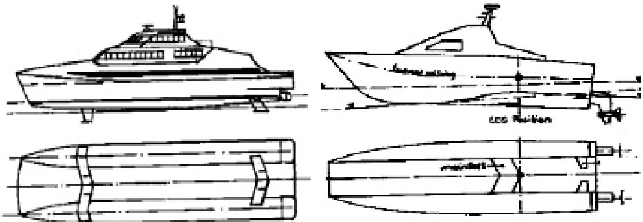
Hình 2.22 Bố trí cánh ngầm cho catamaran
