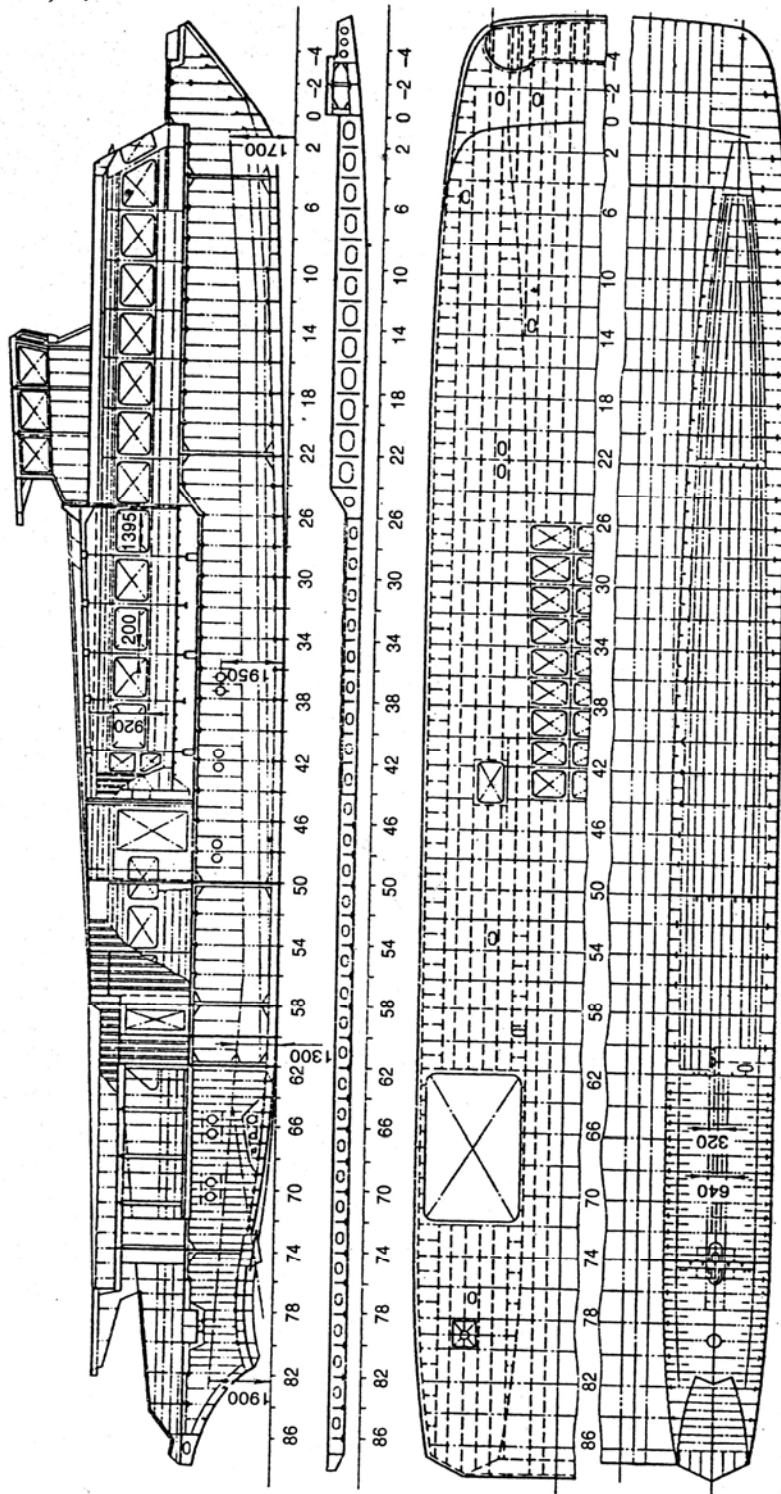
Hình 2.31 Hệ thống kết cấu dọc tàu hai thân
