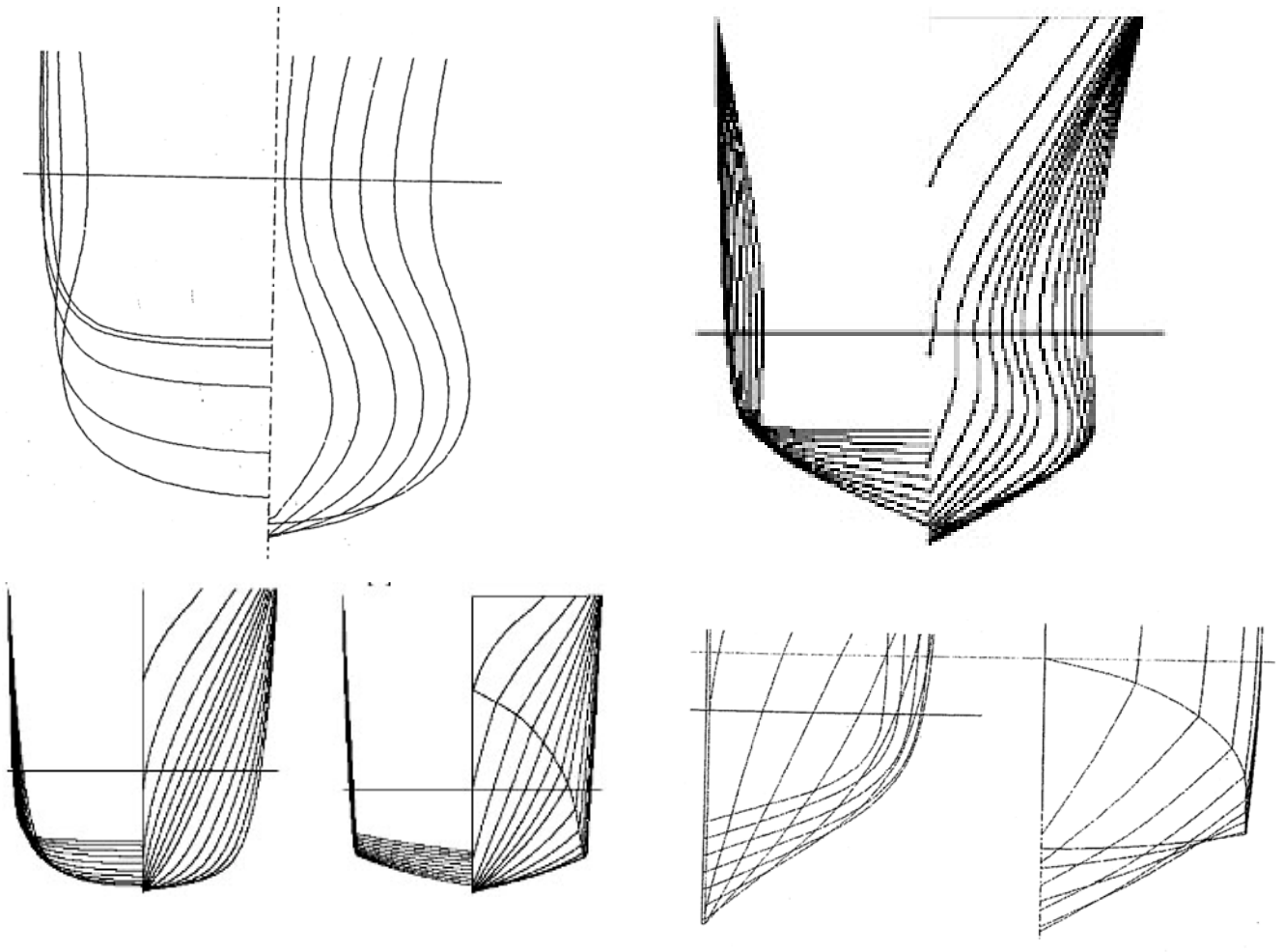
Hình 2.3 Đường hình d0a85c trong tàu hai thân
