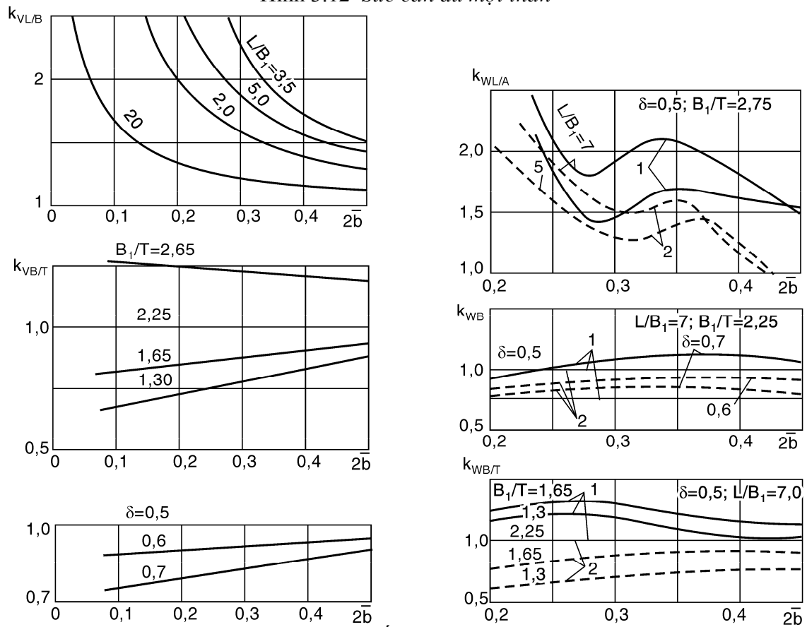
Hình 3.13 Hệ số cản nhớt tàu SWATH
