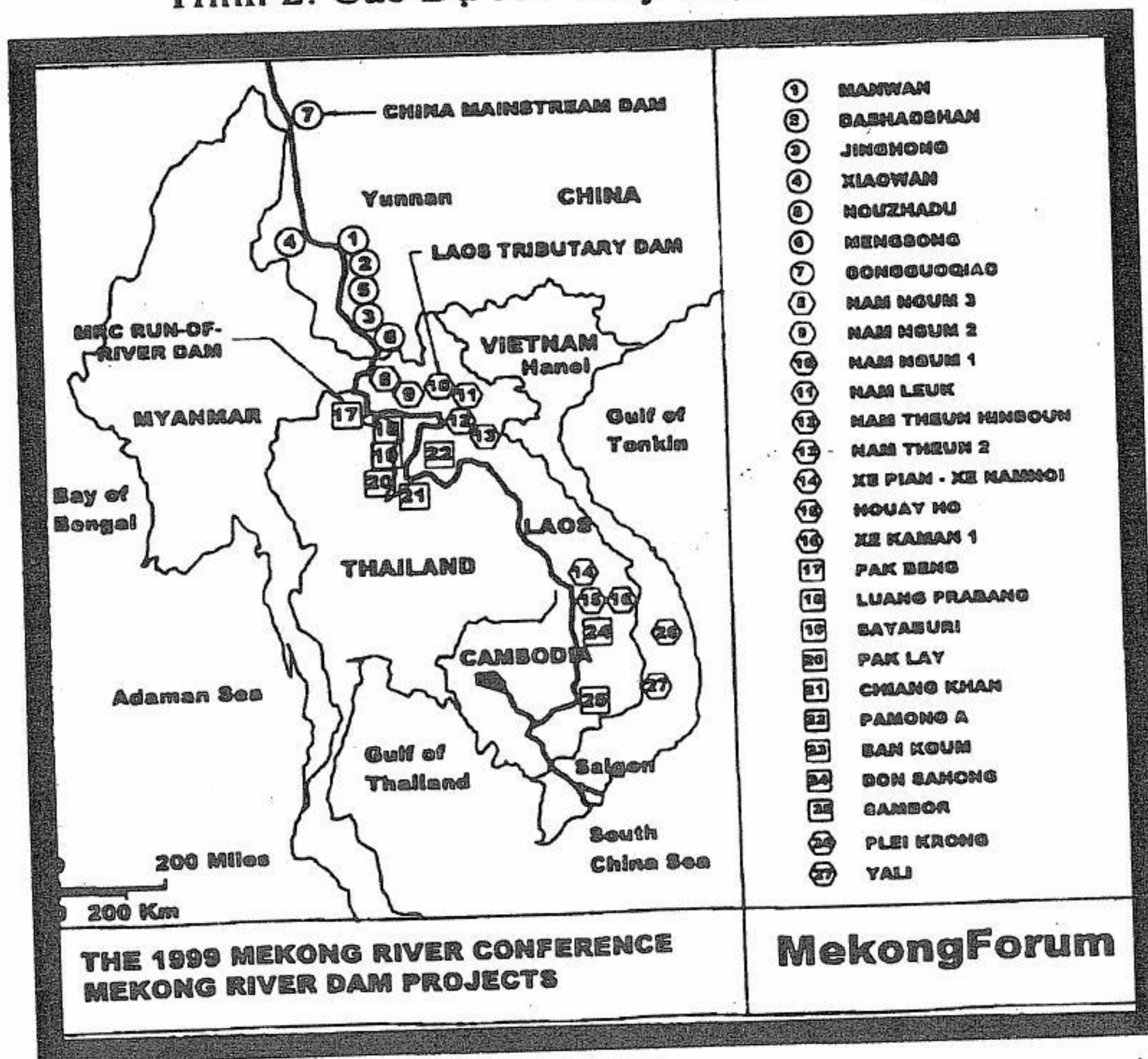
Hình 2: Các Dự Án Thủy Điện Mekong
