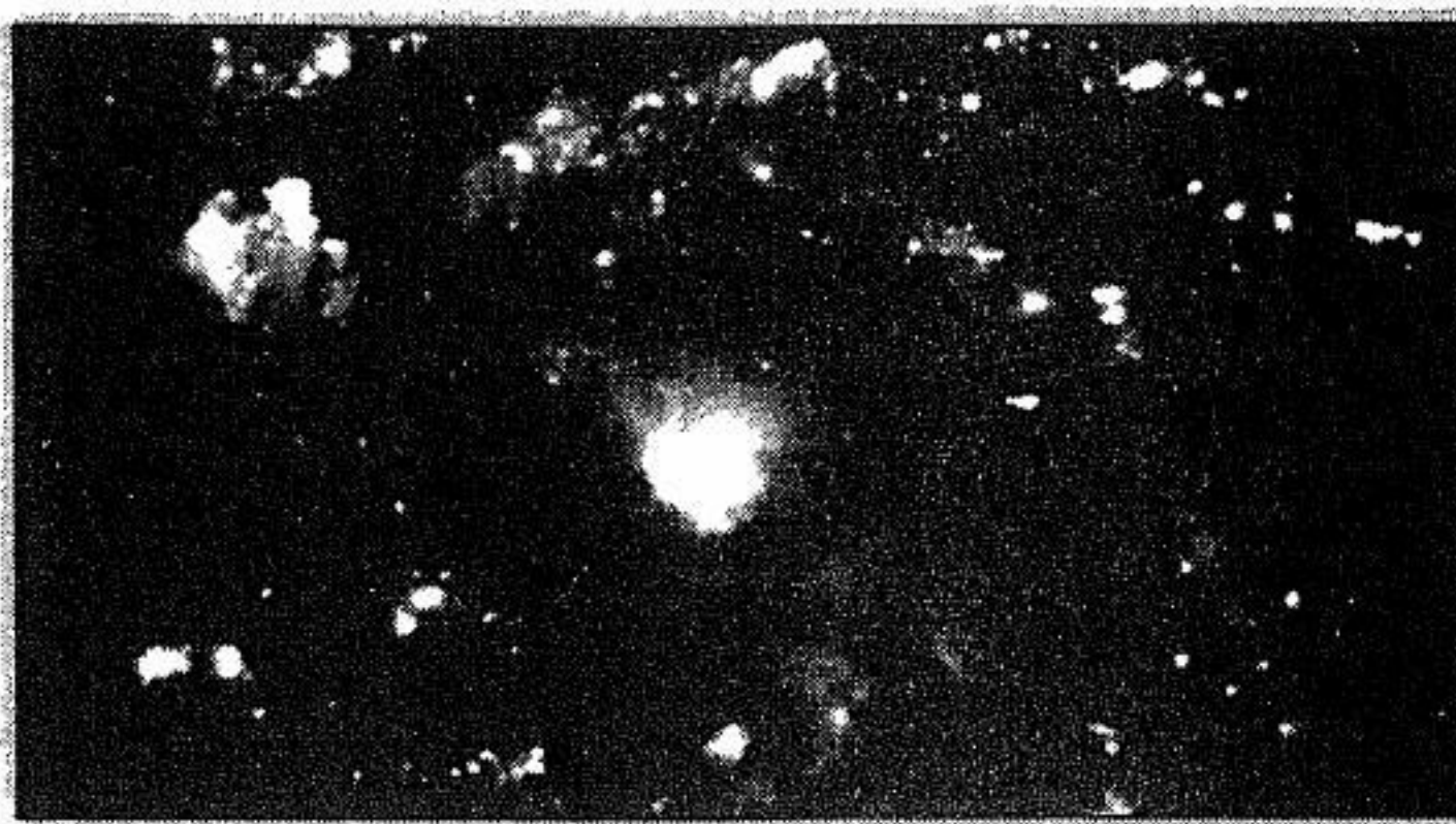
Các galaxy nằm trong bối cảnh của chòm sao Virgo -- theo nghiên cứu của Đại học Indiana. Nhóm nghiên cứu này cho rằng tuổi của vũ trụ có thể chỉ mới...bảy tỉ năm; trong khi nhóm nghiên cứu ở Đại học Harvard lại cho rằng vũ trụ đã được hình thành từ chín tới 14 tỉ năm rồi.
