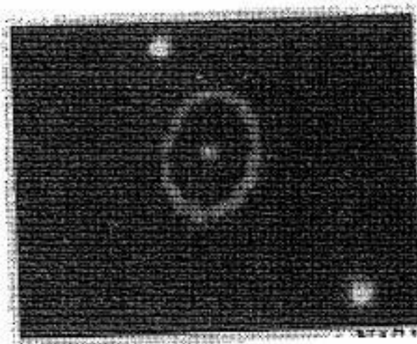
Một siêu sao mới (supernova) đang nổ ở cách trái đất 500 triệu năm ánh sáng. (Nghiên cứu của Đại học Harvard)
