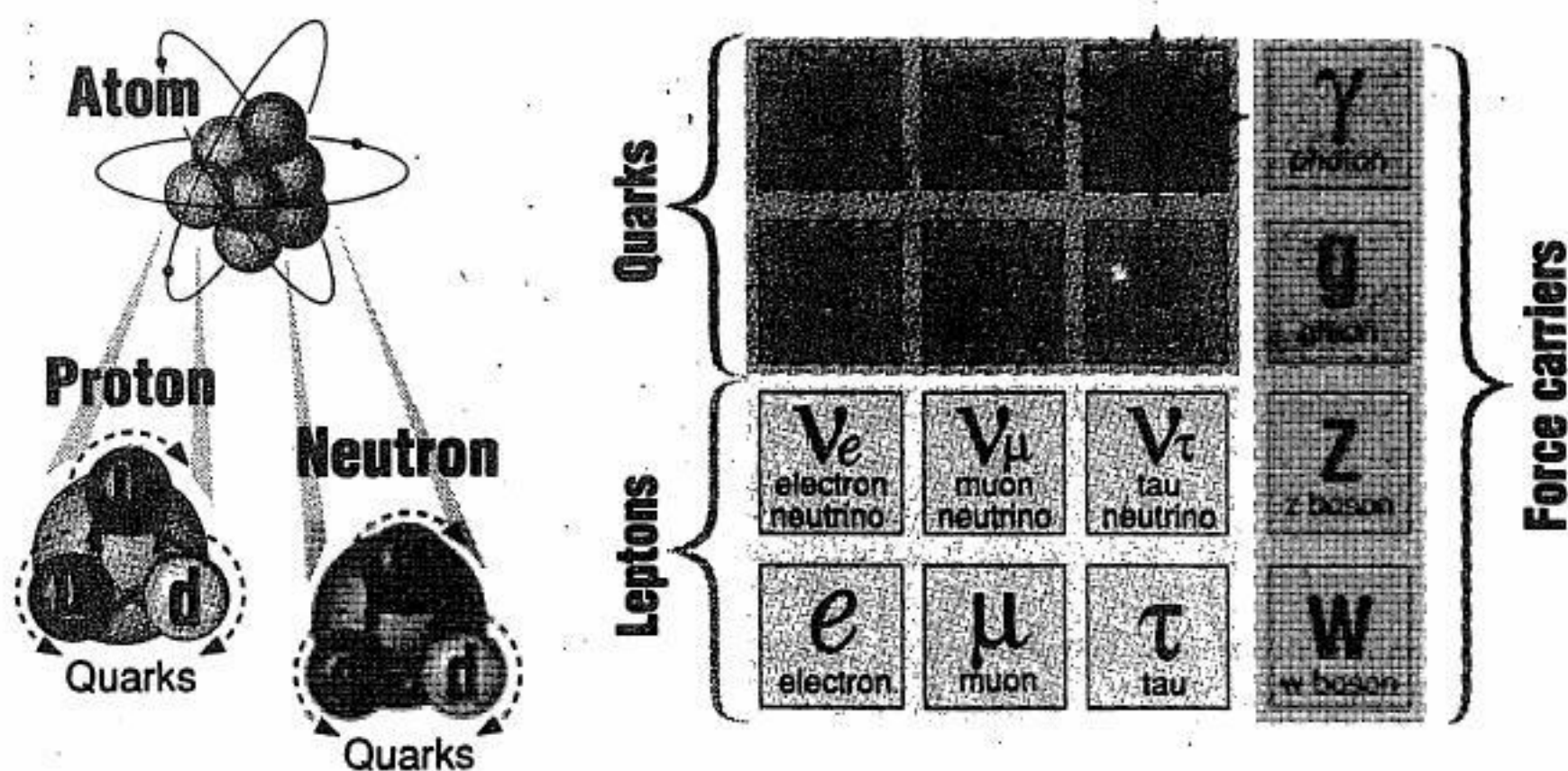
Những vi hạt "quác" trong proton và newtron
