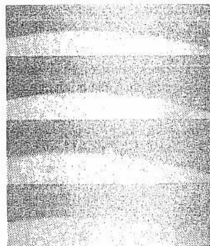
Hình dưới cho thấy các giai đoạn một mảnh sao chổi rớt xuống Mộc Tinh. Hình trên cho thấy dấu vết của sự va chạm - lớn bằng diện tích tiểu bang New Hampshire (Hoa Kỳ).
