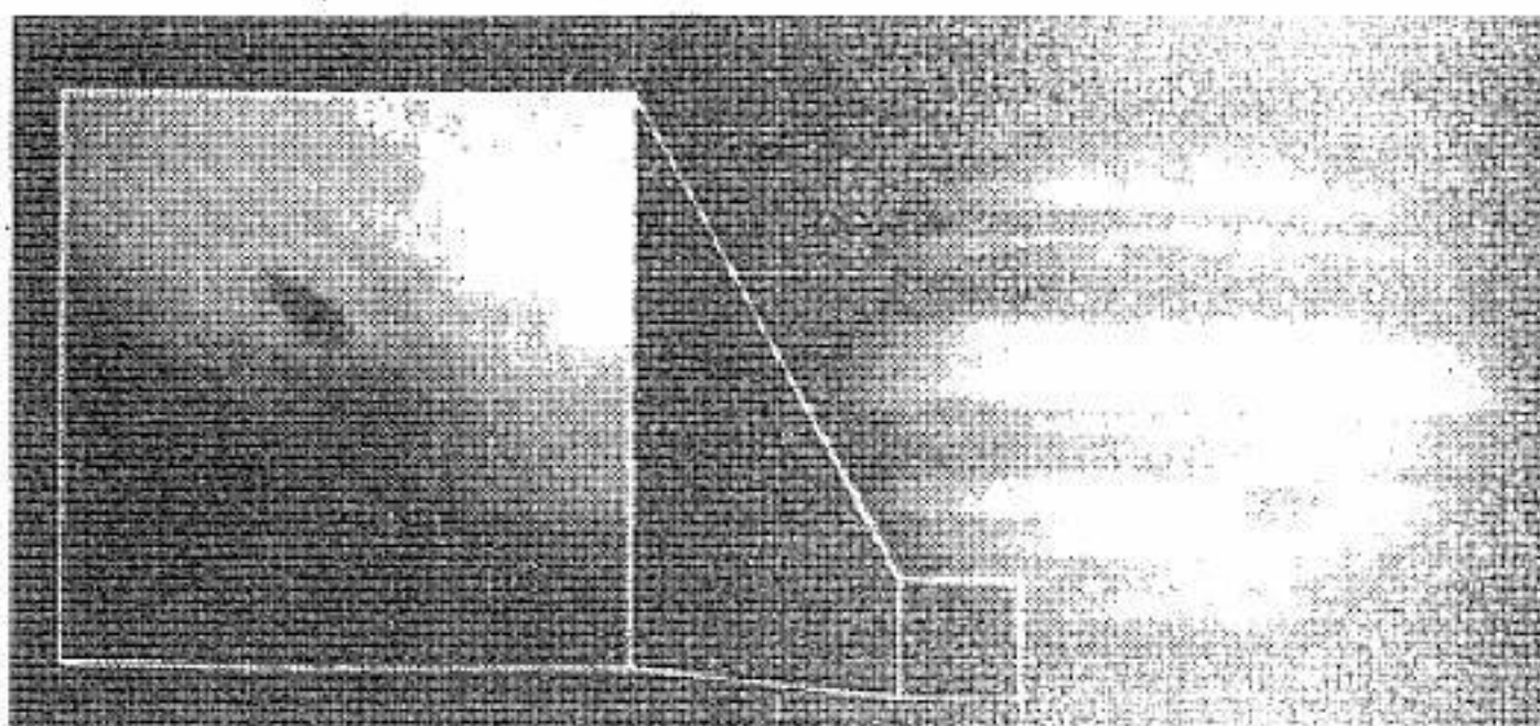
Hình dưới cho thấy các giai đoạn một mảnh sao chổi rớt xuống Mộc Tinh. Hình trên cho thấy dấu vết của sự va chạm - lớn bằng diện tích tiểu bang New Hampshire (Hoa Kỳ).
