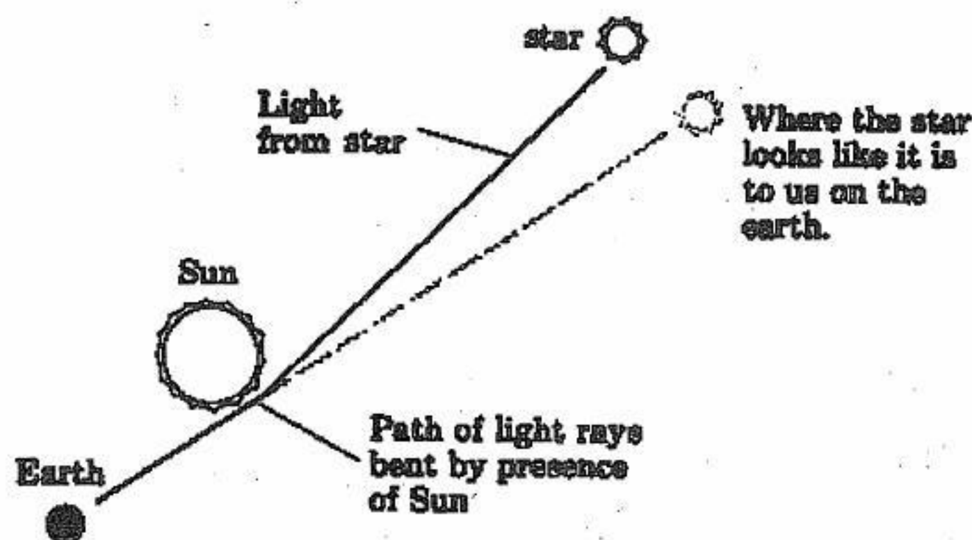
Hình 2 Ánh sáng của ngôi sao bị cong đi khi chạy sát khối lượng Mặt Trời
