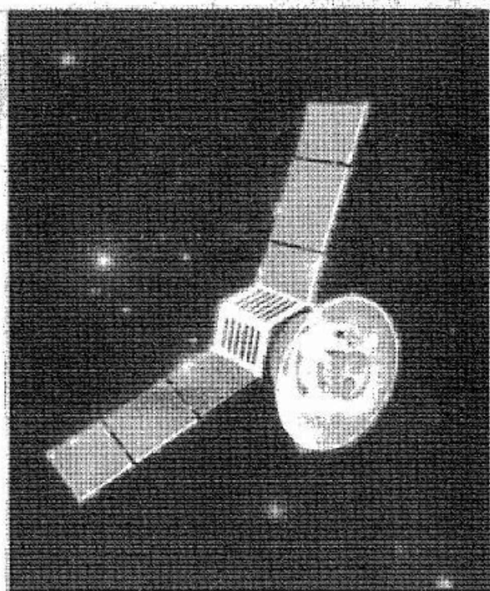
Vệ tinh COBE thám sát bức xạ hóa thạch trong vũ trụ.
