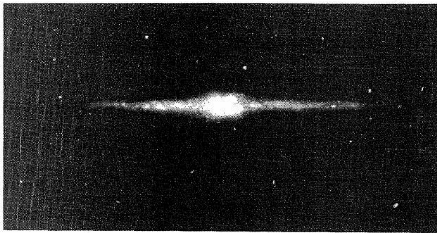
Hình ảnh một galaxy chụp theo chiều nằm.
