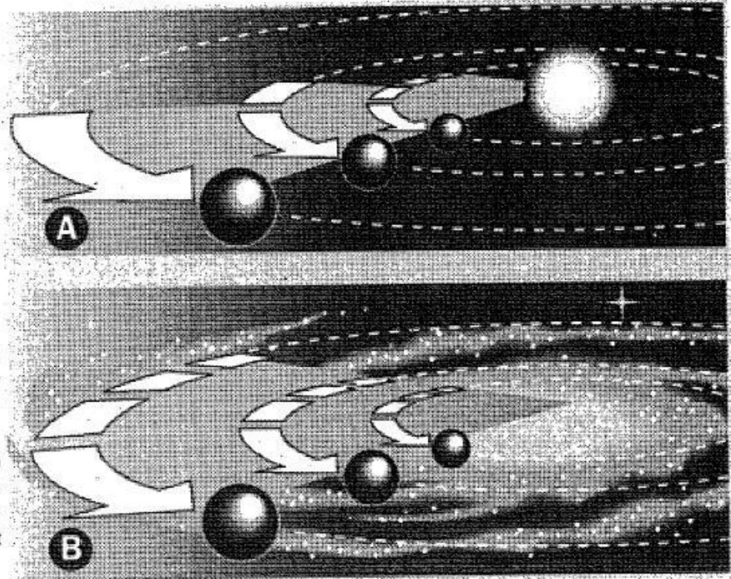
Hình A: Các hành tinh quay xung quanh Mặt Trời, theo đúng luật Newton, hành tinh ở gần Mặt Trời quay nhanh, hành tinh ở xa quay chậm.
