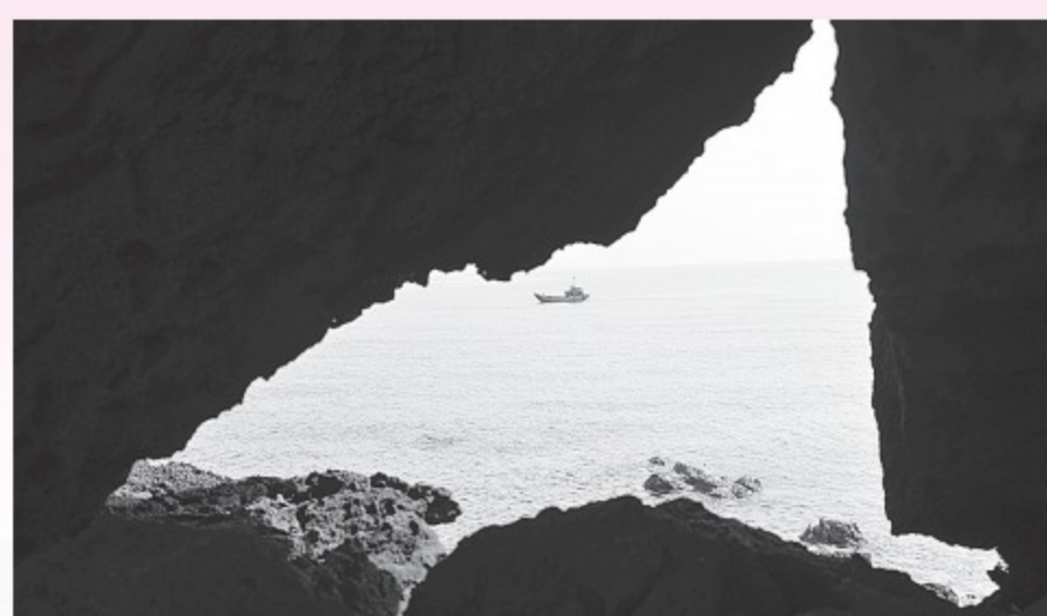
Một khối nham thạch ở bãi sau (đảo Bé, Lý Sơn)
