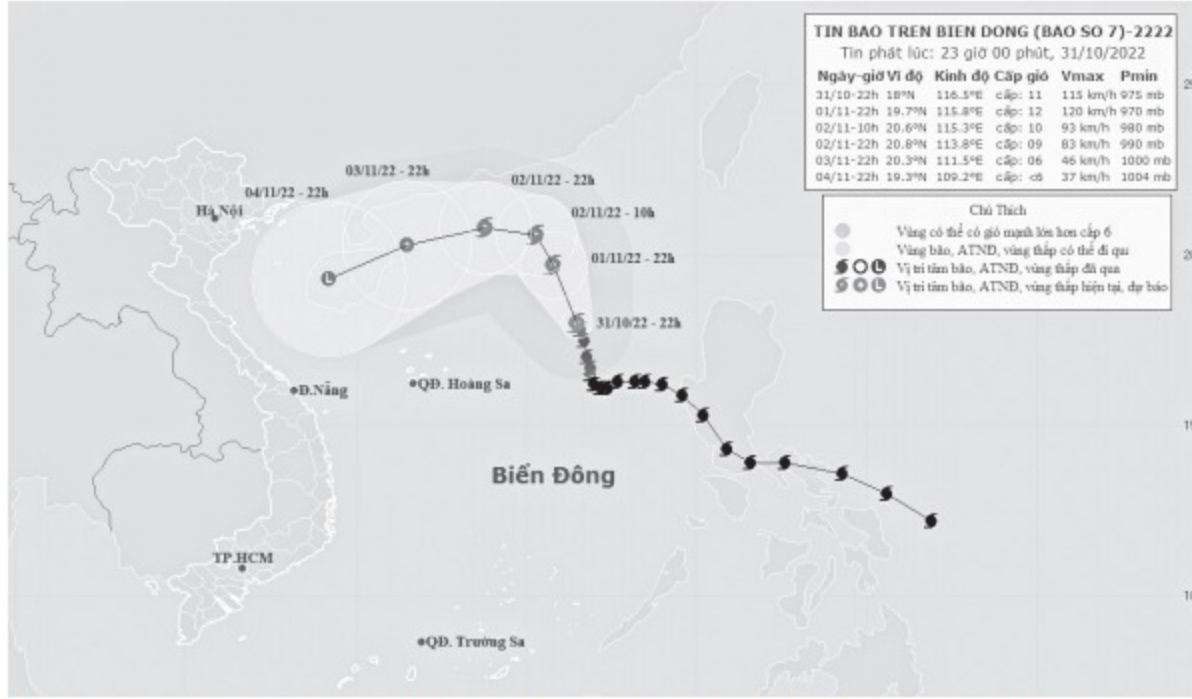
Dự báo đường đi của bão số 7, cập nhật lúc 23 giờ ngày 31.10 NGUỒN: TRUNG TÂM DỰ BÁO KHÍ TƯỢNG THỦY VĂN QUỐC GIA
