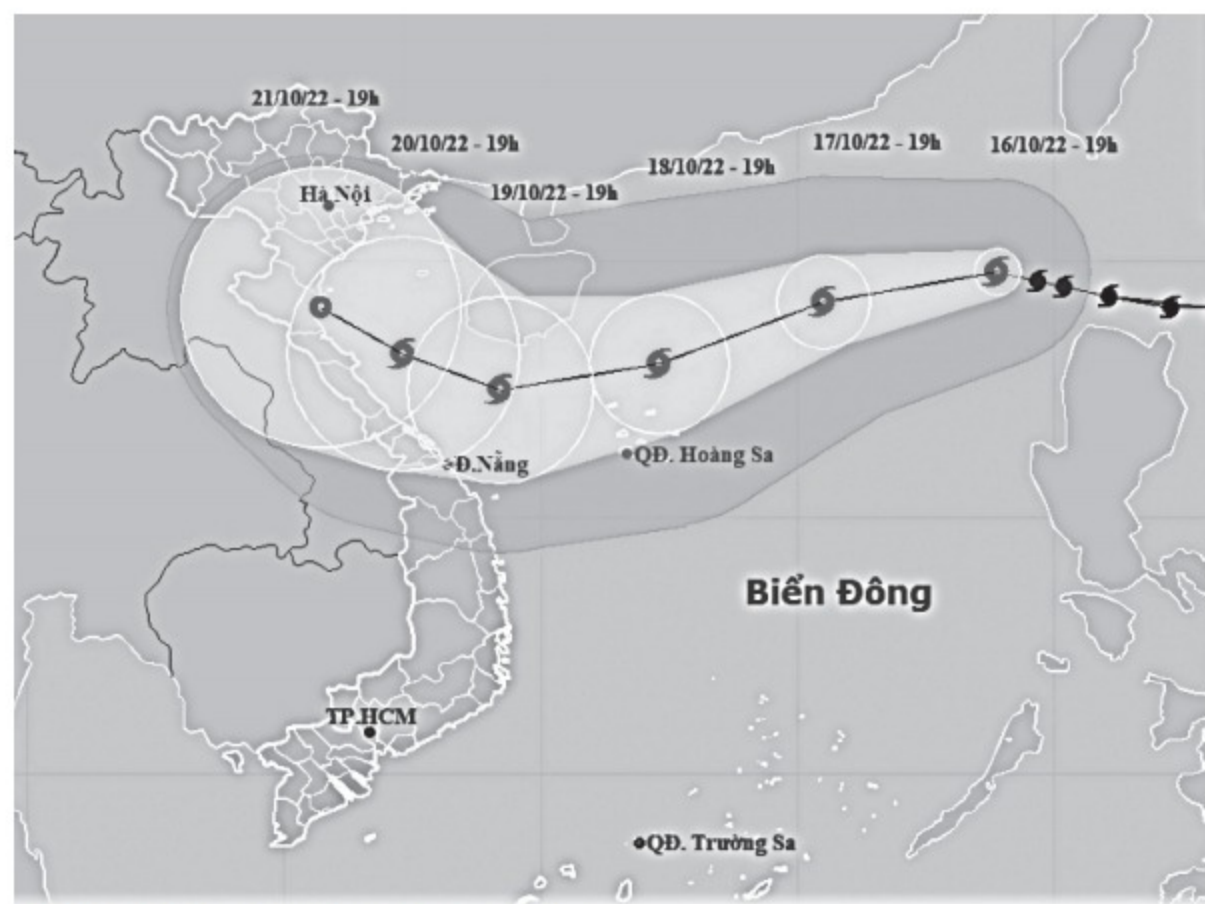
Dự báo hướng đi của bão số 6 NGUỒN: TRUNG TÂM DỰ BÁO KHÍ TƯỢNG THỦY VĂN QUỐC GIA
