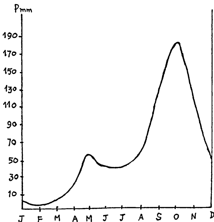
Bảng chỉ sự biến-thiên vũ-lượng tại đồng-bằng PHAN-RANG
