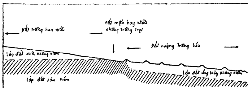
Sơ đồ chỉ rõ sự liên hệ giữa tính chất kiềm và mền trong đất với các loại đất ở Phan-Rang.
