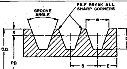
BẢNG 7 : KÍCH THƯỚC RÃNH VÀ DUNG SAI CHO RÒNG RỌC NHIỀU ĐAI V
