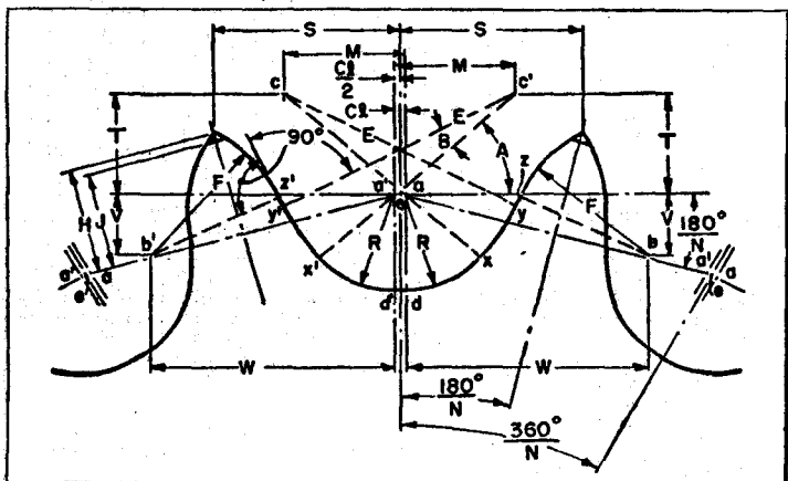
BẢNG 9 : DẠNG RĂNG ĐĨA TIÊU CHUẨN MỸ CHO XÍCH LĂN Table 9. AMERICAN STANDARD SPROCKET TOOTH FORM FOR ROLLER CHAIN (ASA B29.1-1957)
