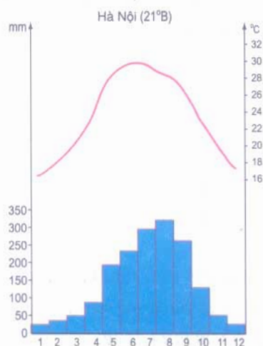
Hình 7.3 - Biểu đồ nhiệt độ và lượng mưa của Hà Nội
