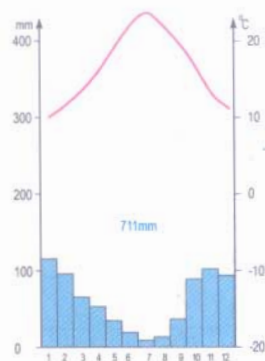
Hình 58.2 - Biểu đồ nhiệt độ và lượng mưa ở Pa-ler-mô (I-ta-li-a)
