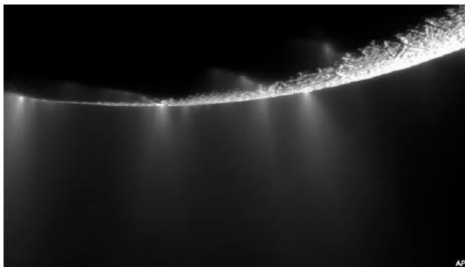
Ảnh của cơ quan NASA chụp cho thấy các tia hơi nước bốc lên từ cực nam của mặt trăng Enceladus của Sao thổ
