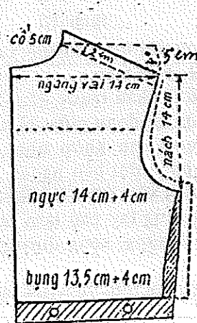
Thân sau Hình 27c
