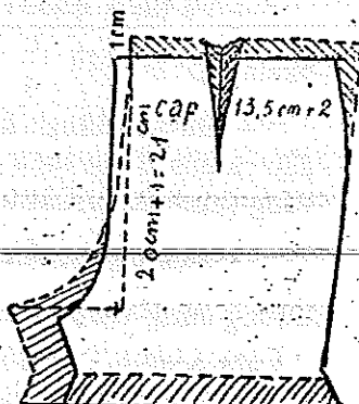
Thân sau (theo dấu chấm)
