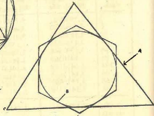
A Tam-giác đều ngoại-tiếp
