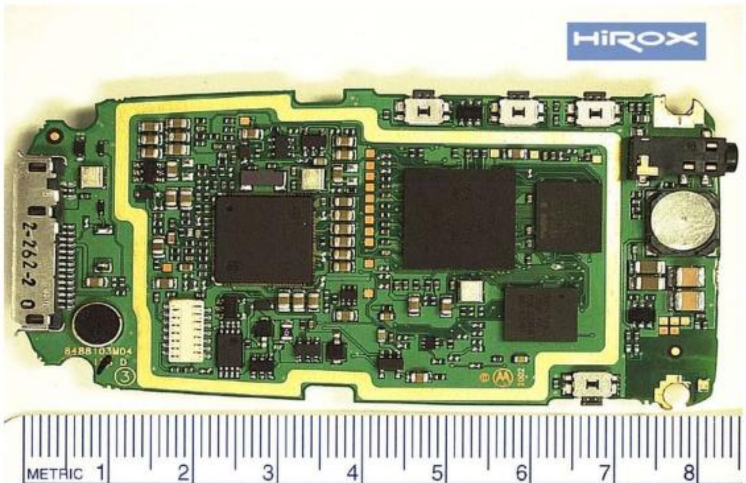
Bên trong điện thoại cầm tay ngày nay (Theo http://www.hirox-usa.com ).
