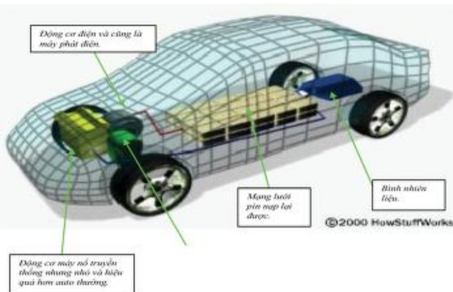
Cấu trúc Auto Hybrid kiểu song song (Theo www.howstuffworks.com)
