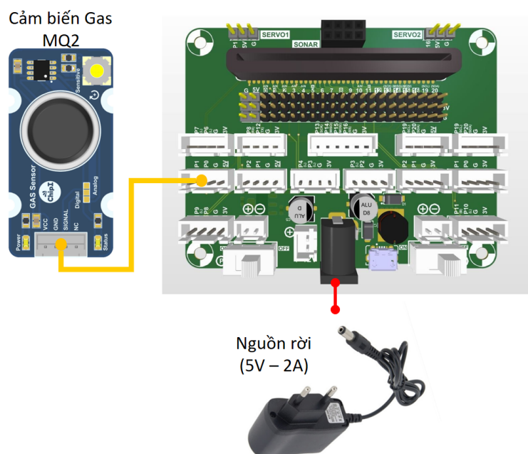
Hình 10.3: Kết nối với cảm biến khí Gas MQ2
