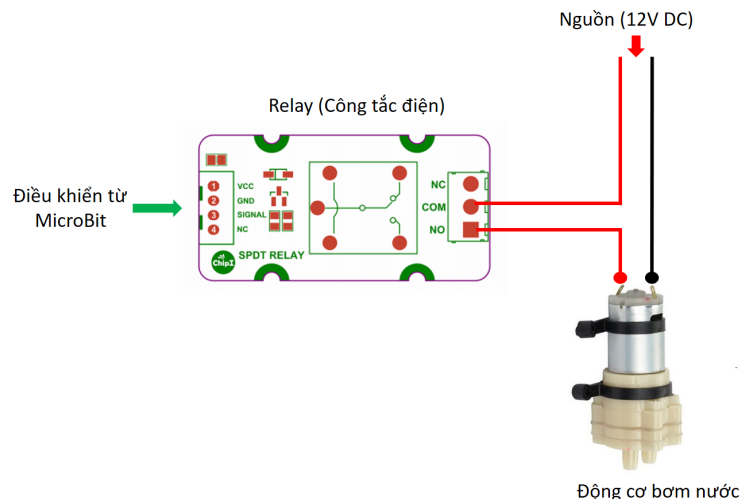
Hình 8.2: Kết nối Relay và Máy bơm
