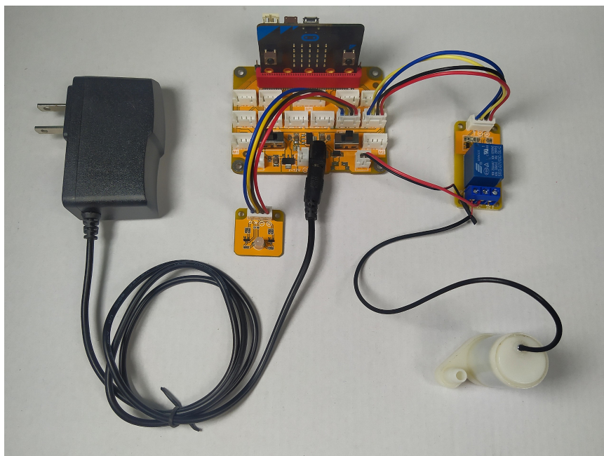
Hình 8.3: Kết nối mạch điện cho hệ thống
