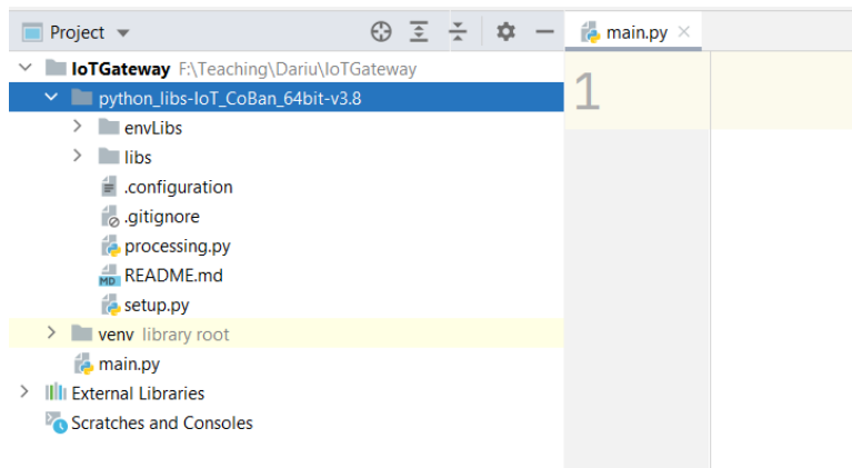
Hình 3.12: Thư viện đã được thêm vào dự án
