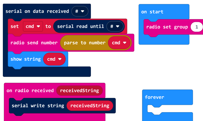
Hình 7.2: Chương trình cho mạch Microbit trung tâm
