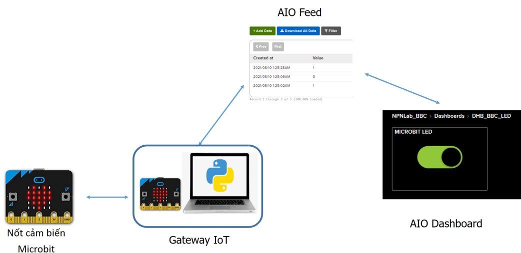
Hình 3.1: Kiến trúc 4 thành phần trong ứng dụng IoT
