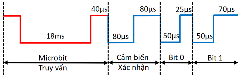
Hình 9.4: Nguyên lý giao tiếp với DHT11
