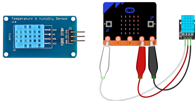
Hình 9.2: Kết nối với DHT11 bằng 3 chân tín hiệu
