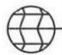
Miura ori
