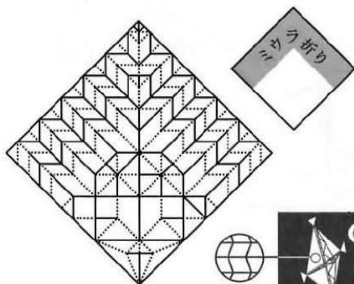
Miura ori
