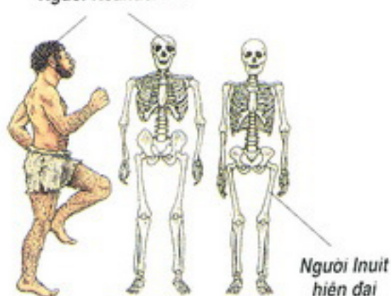
Người Neanderthal
