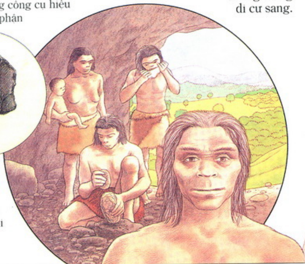
Người Neanderthal
