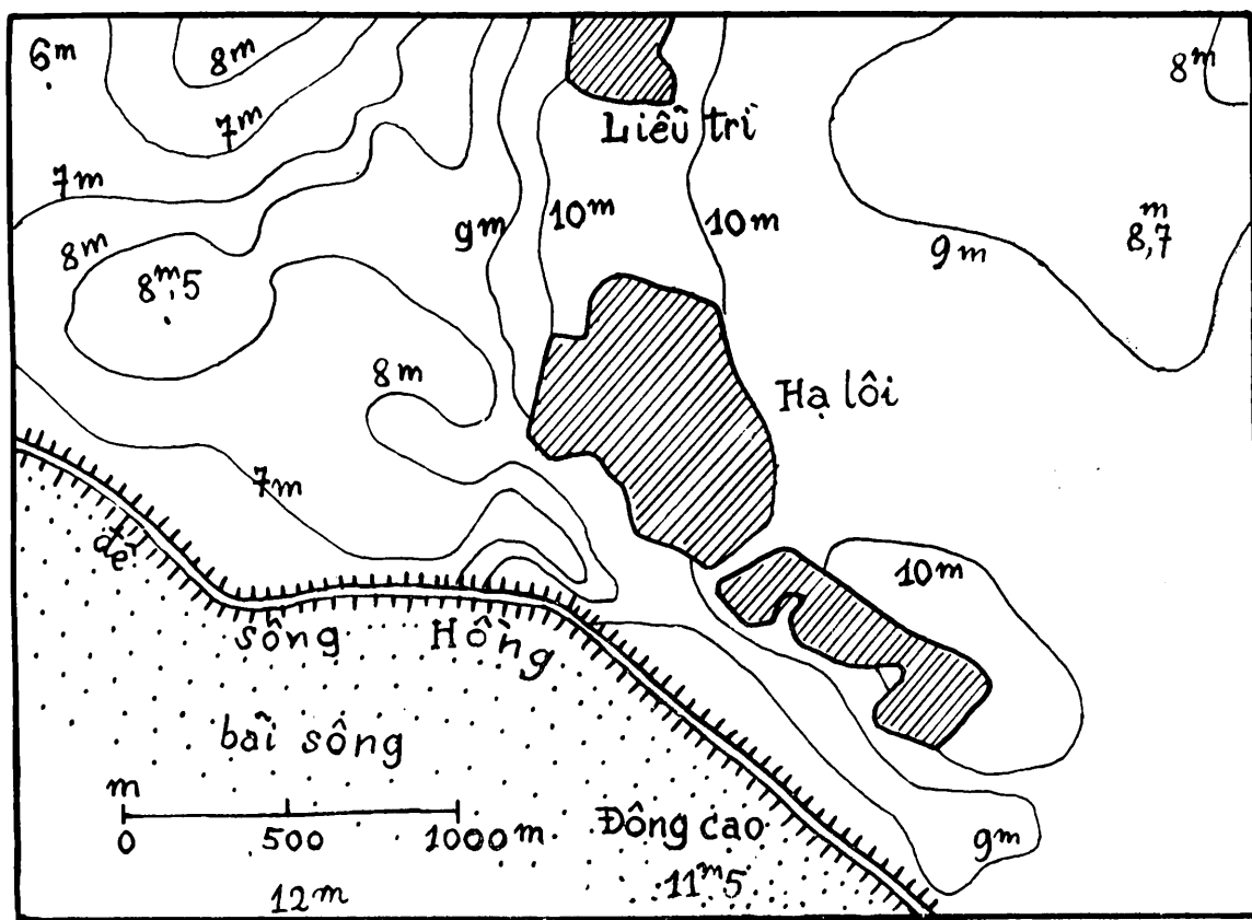
Hình 1 — Lược đồ địa hình vùng Hạ-lôi, thuộc xã Mê-linh, huyện Yên-lãng, tỉnh Vĩnh-phú. Phần kẻ chéo là làng xóm, phần chấm chấm là bãi sông. Các đường đẳng cao cách nhau 1m chiều cao. Trong phần bãi sông không vẽ các làng xóm và đường đẳng cao, chỉ ghi một vài điểm cao đáng chú ý của các gờ sông ngày nay.
