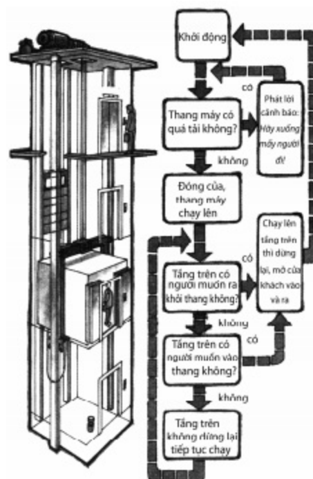
Sơ đồ vận hành của thang máy
