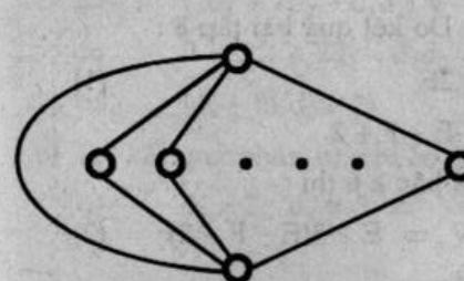
K_{1,1,r}
