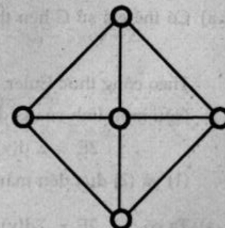
K_{1,2,2}
