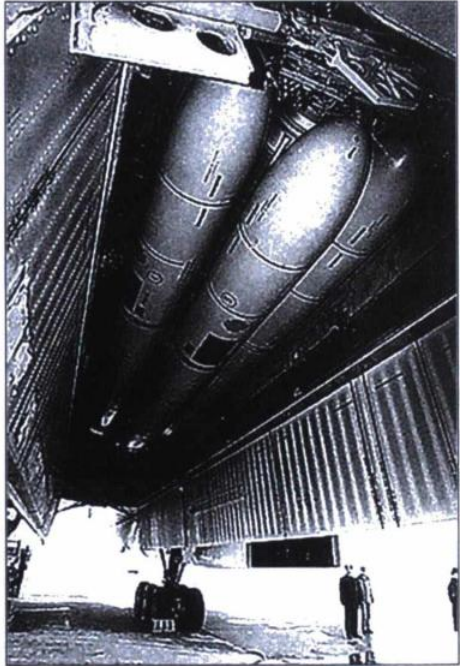
Tên lửa KH-55 Granat có thể mang đầu đạn hạt nhân được lắp đặt trong khoang máy bay ném bom chiến lược Tu-160
