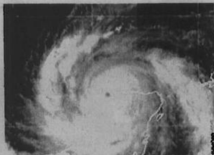
Bão Isidore, nhìn từ vệ-tinh
