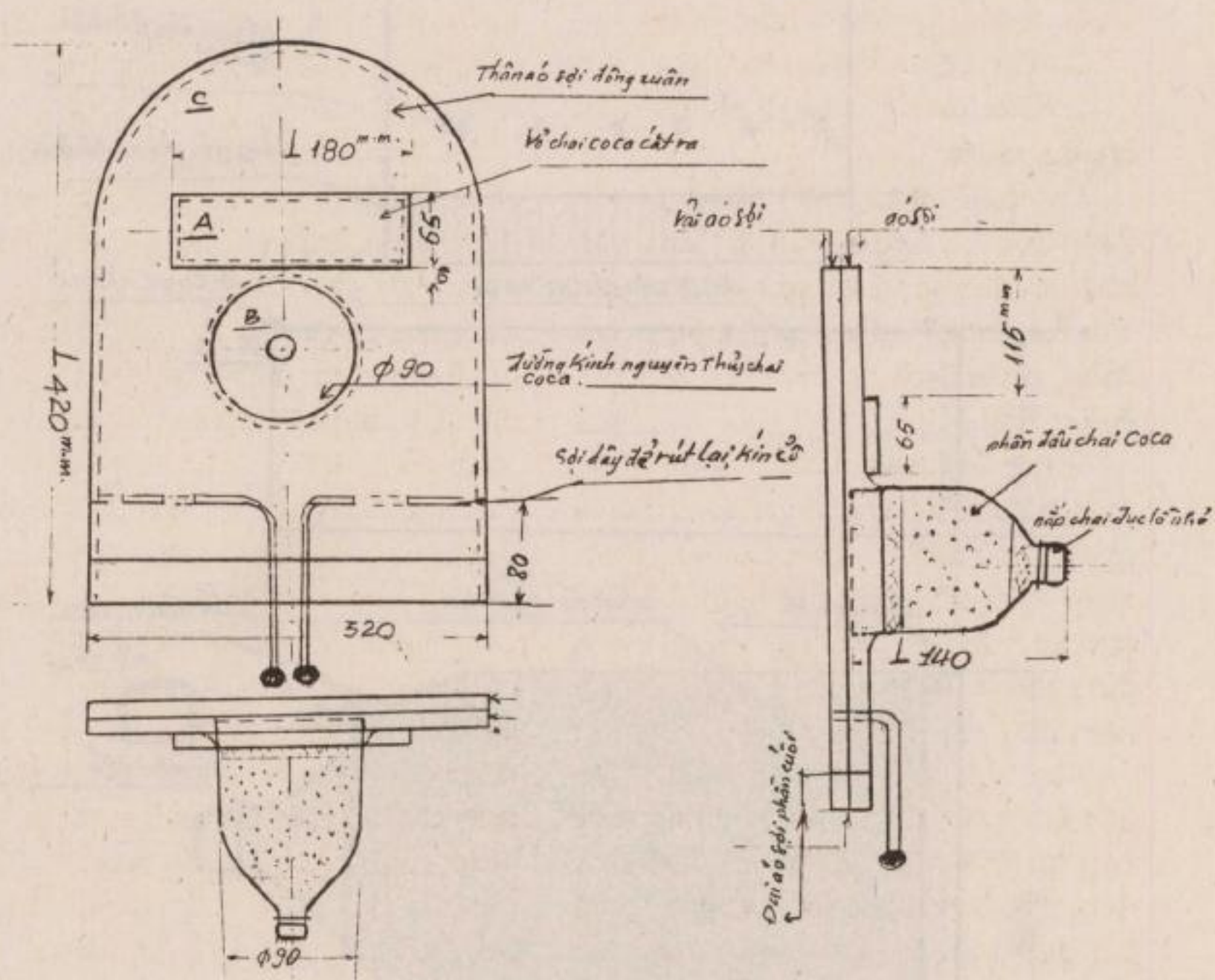
Bản vẽ 1: Qui-trình công-nghệ chế-tạo mũ chống hơi cay (kích-thước: tính bằng mm)
