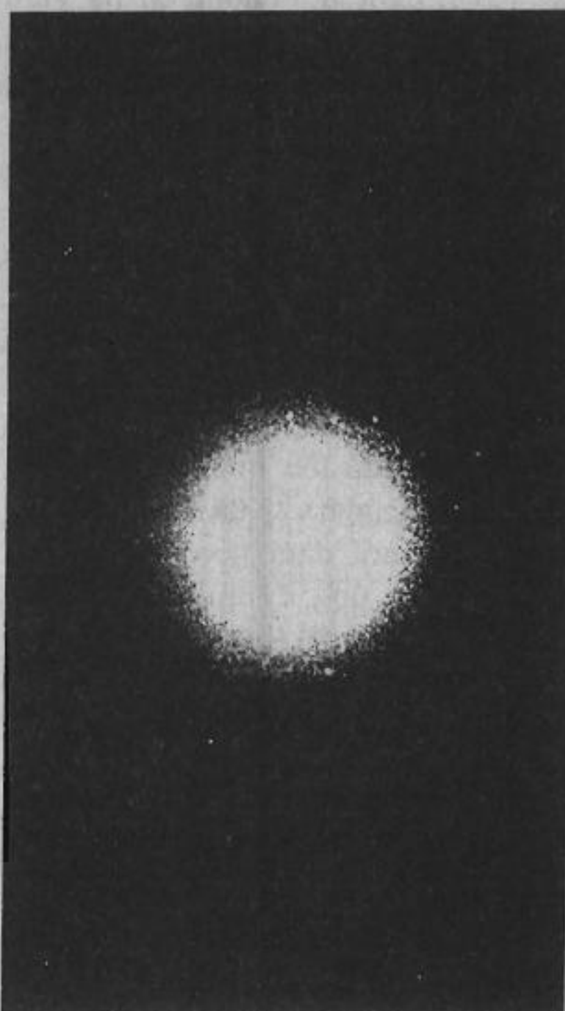
Hình-ảnh rõ-ràng nhất về quái-vật vũ-trụ, tức thiên-hà M87, lúc chưa và lúc black hole tác-động làm phóng-xuất với năng-lượng, tức là luồng hạt lốc xoáy đi ra bằng tốc-độ ánh-sáng, phóng xa đến 6.000 quang-niên, cách trái đất 50 triệu quang-niên.
