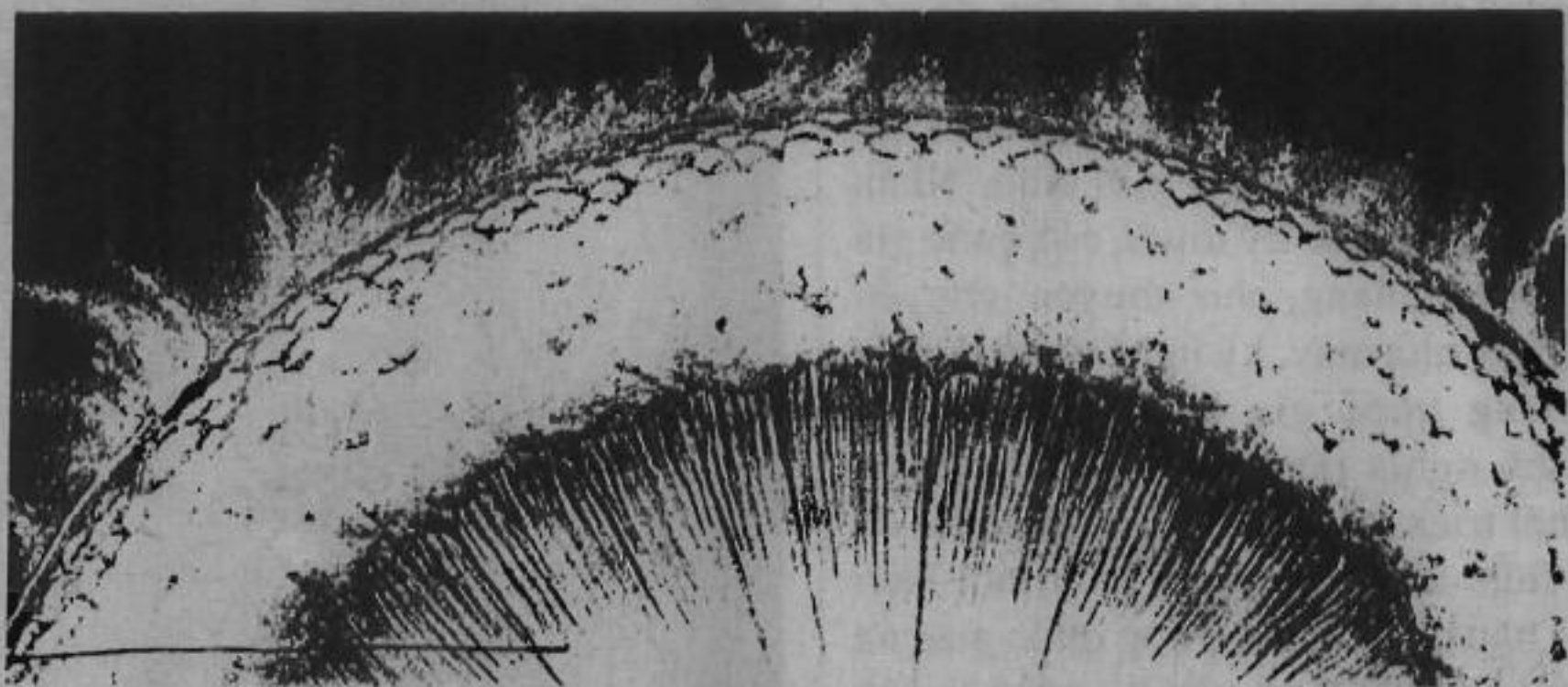
Phản-ứng hạt nhân liên-tục trong lõi mặt trời, cung-cấp năng-lượng cho lớp vỏ ngoài biến-hóa Deuterium (hydrogen nặng) thành Helium, thải bớt vật-chất ra ngoài không-gian bằng các tia vũ-trụ (gió mặt trời).
