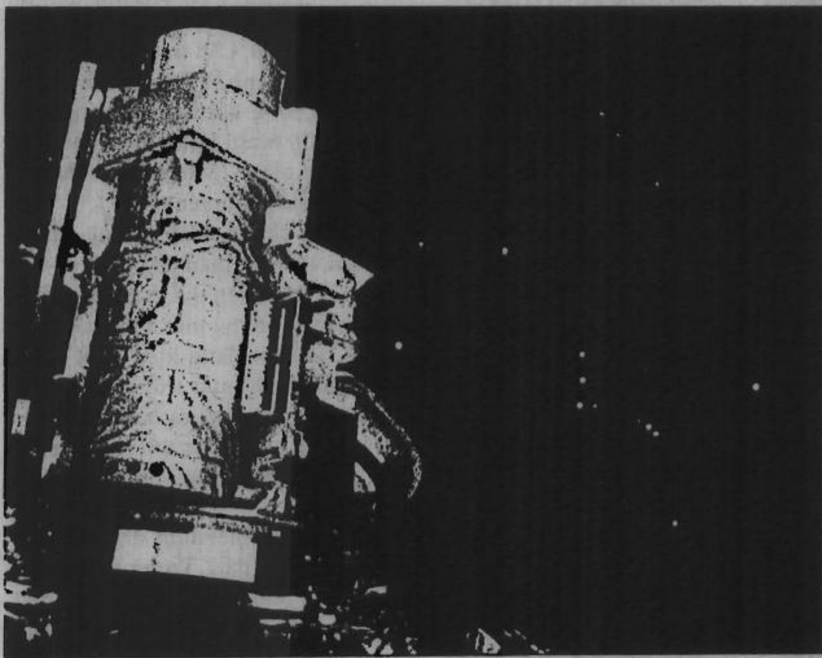
Chòm sao Orion chụp từ phi-thuyền vũ-trụ (hình trên), và qua hình vẽ (xem trang trước). Sao hồng đại khổng-lồ nằm ở vai phải hiệp-sĩ (sao Betelgeuse). Sao xanh khổng-lồ Rigel ở vị-trí chân trái.
