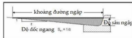
Thiết đồ mặt đường với độ ngập
