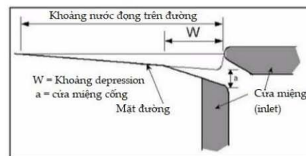
Thiết đồ cửa miệng cống (gutter) của lộ đường
