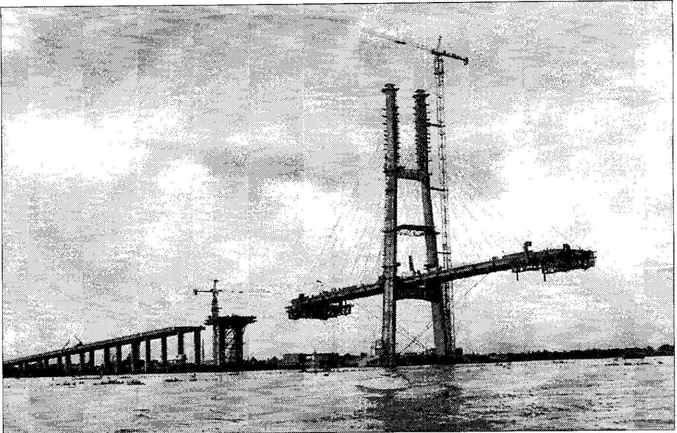
Cầu Mỹ Thuận đang xây cất.
