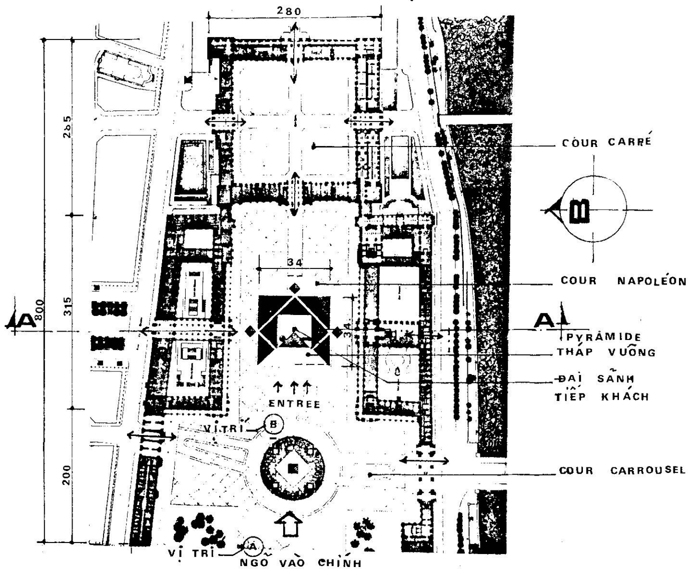
BÌNH ĐỒ TRỆT
