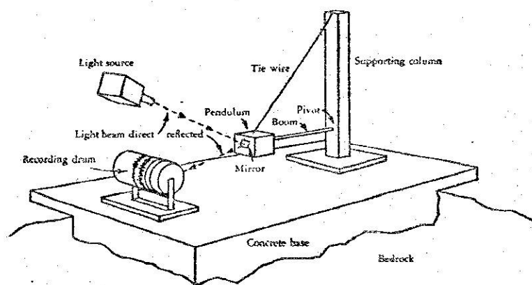
CHÂN ĐỘNG KÝ VÀ CÁC LẦN SÓNG CHÂN ĐỘNG CHI NHẬN ĐƯỢC
