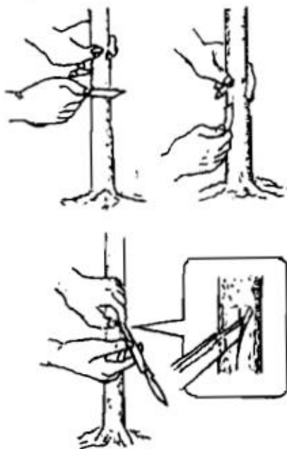
Hình 38: Mở miệng ghép mầm
