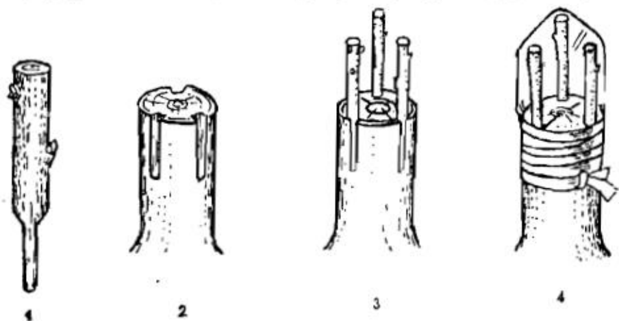
Hình 67: Ghép nêm
