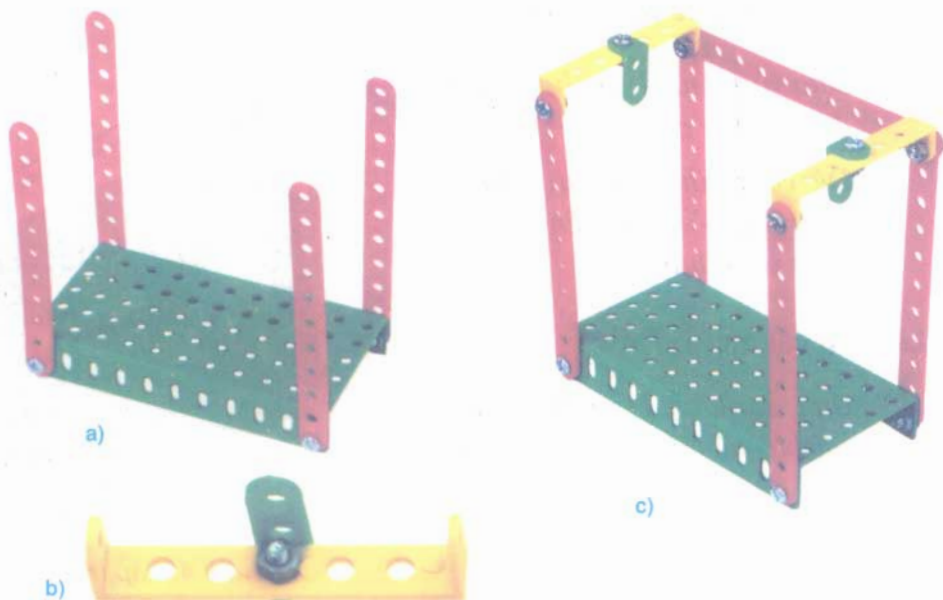
Hình 2. Lắp giá đỡ trực đu
