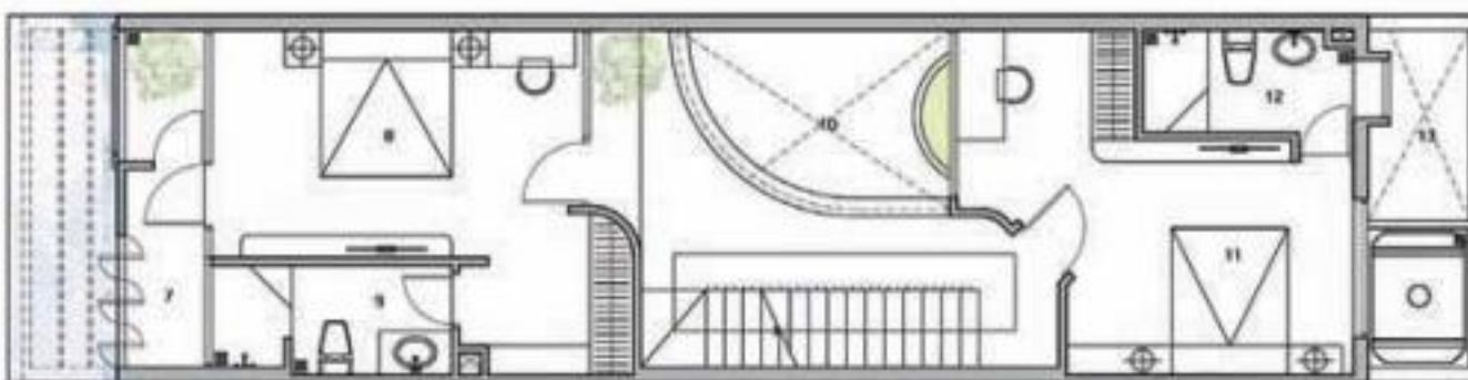
Mặt bằng trệt
