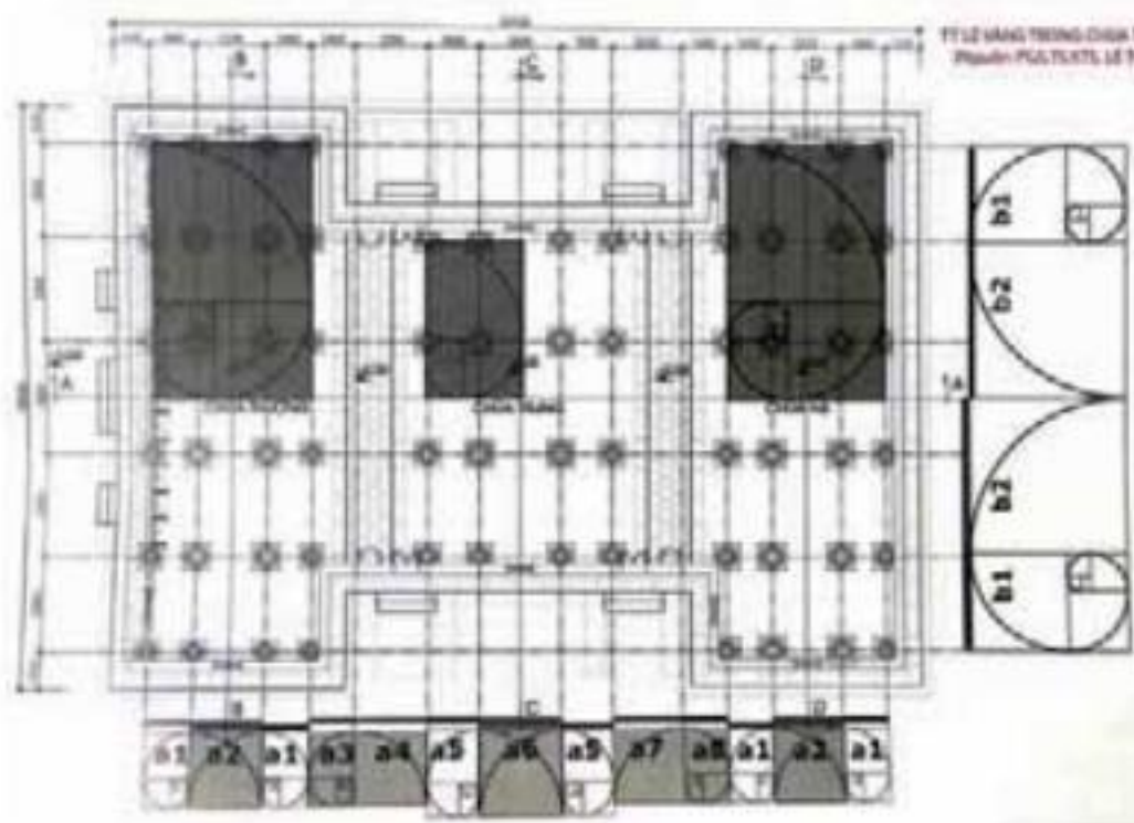
Bảng nghiên cứu kích thước kiến trúc cổ truyền Việt Nam với tỷ lệ vàng kiến trúc Tây phương
