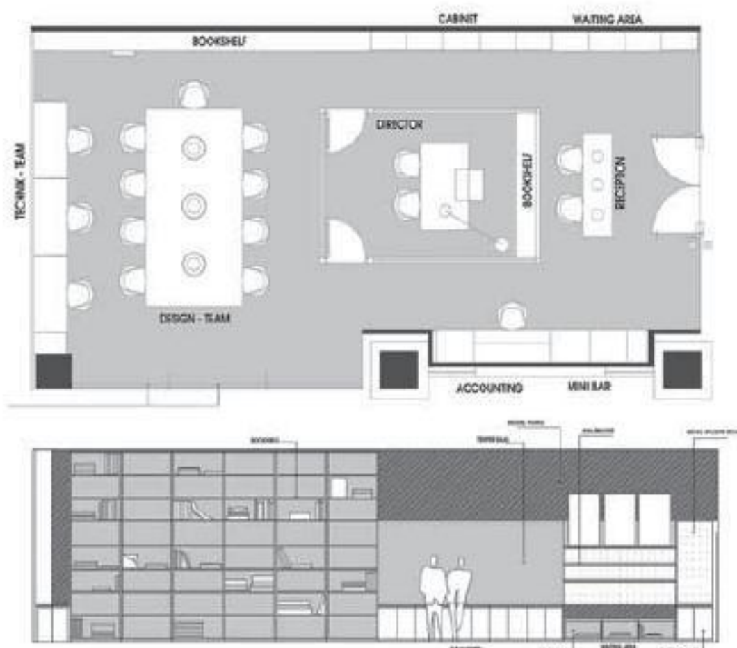
Mặt bằng bố trí
