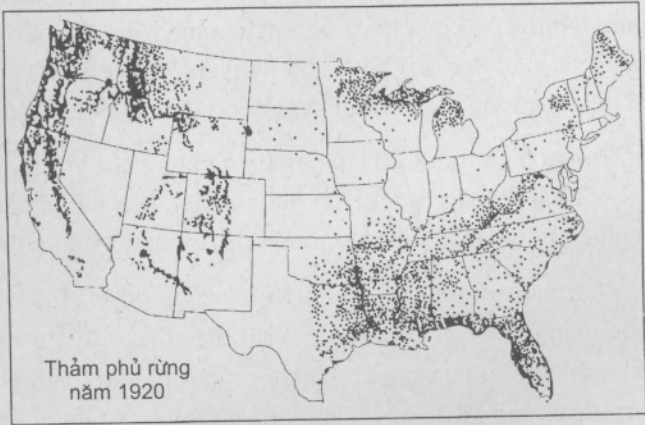
Hình 47. Phân bố rừng tự nhiên ở Mỹ năm 1620 và 1920.
