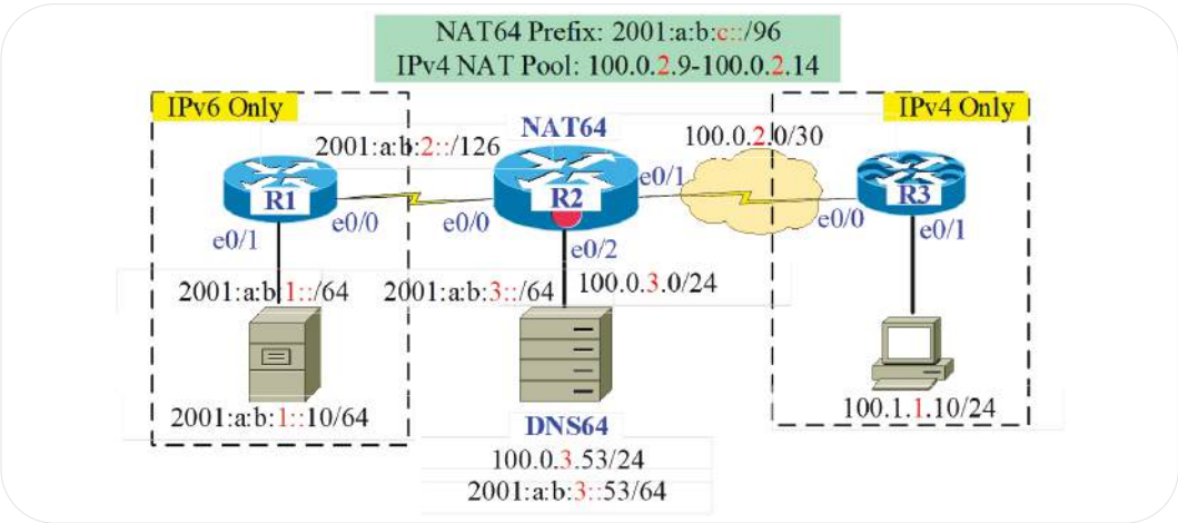
Hình 133. Mô hình LAB IPv6 Only với NAT64 và DNS64 độc lập
