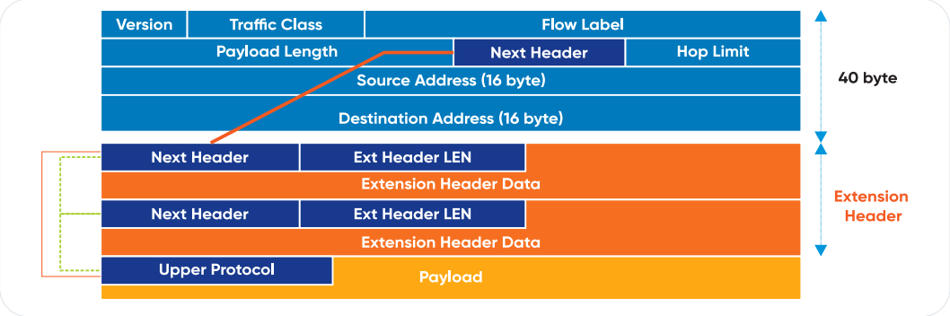
Hình 27. Vị trí của Extension Header
