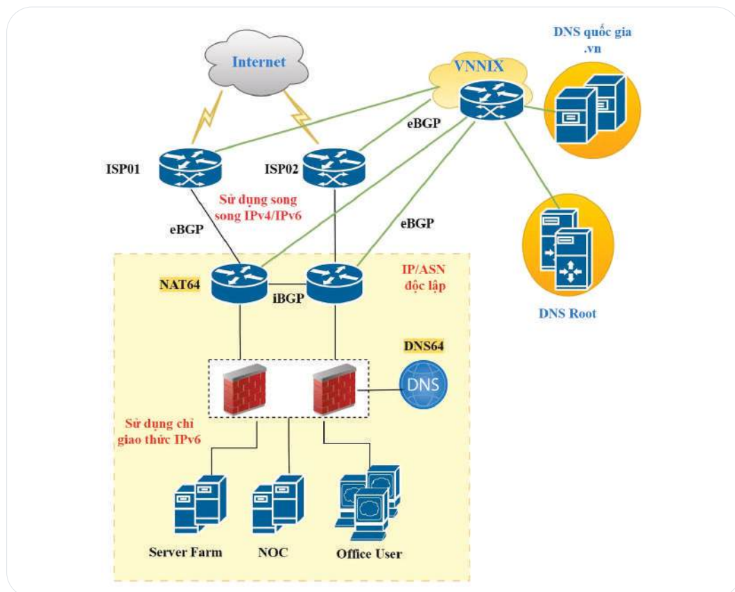
Hình 132. Mô hình mạng hiện đại với IP/ASN độc lập và kết nối đa hướng
