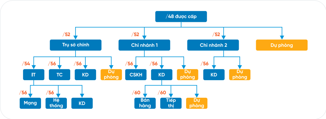
Hình 107. Minh họa việc phân tầng và phân bổ Prefix Length cho một doanh nghiệp
