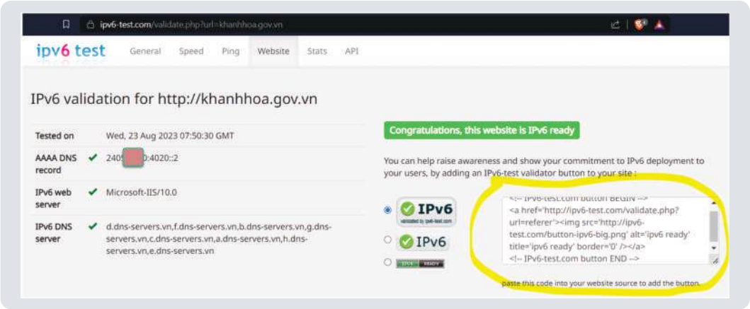
Hình 175. Kiểm tra máy chủ dịch vụ khanhhoa.gov.vn
