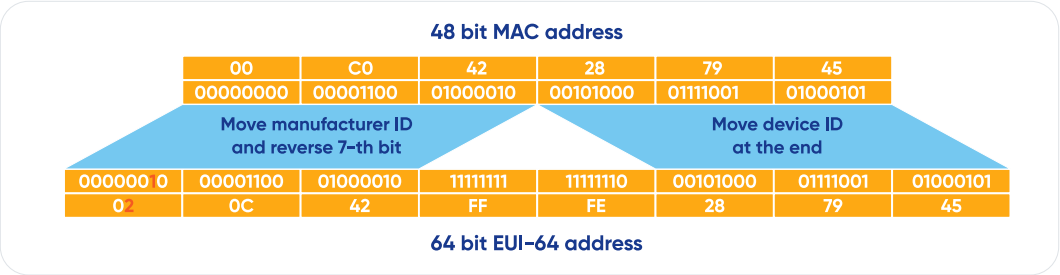
Hình 77. Chi tiết nguyên tắc của EUI-64
