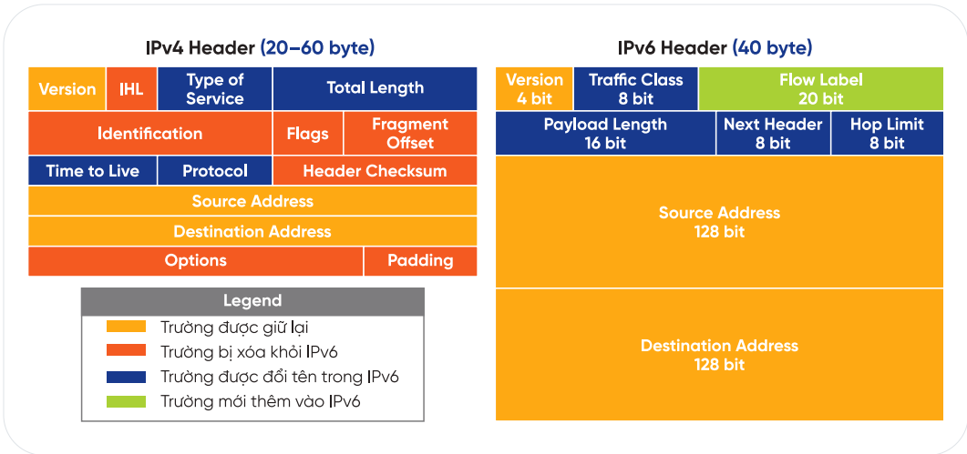
Hình 25. Chi tiết các trường của IPv6
