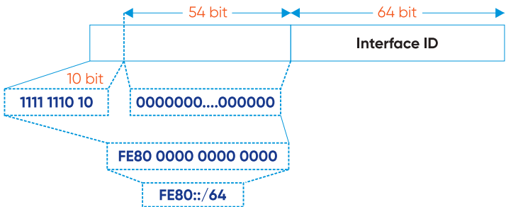
Hình 39. Cấu trúc của địa chỉ LLA
