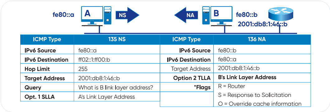
Hình 80. Các bản tin trong kỹ thuật phân giải địa chỉ MAC và IPv6
