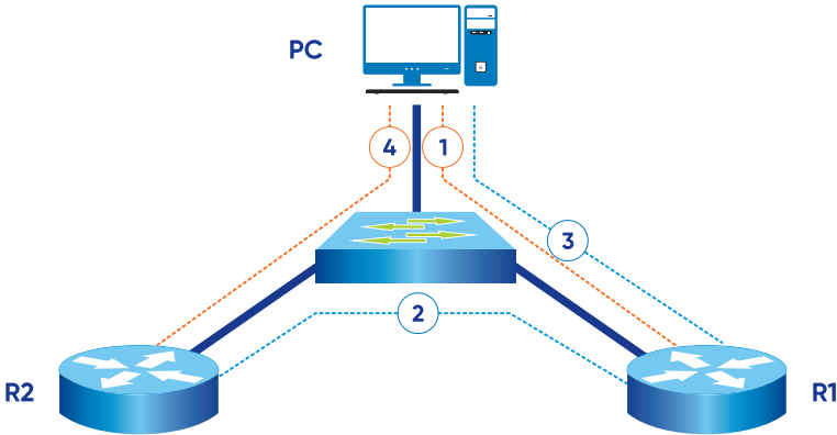
Hình 59. Hoạt động của bản tin ICMP Redirect
