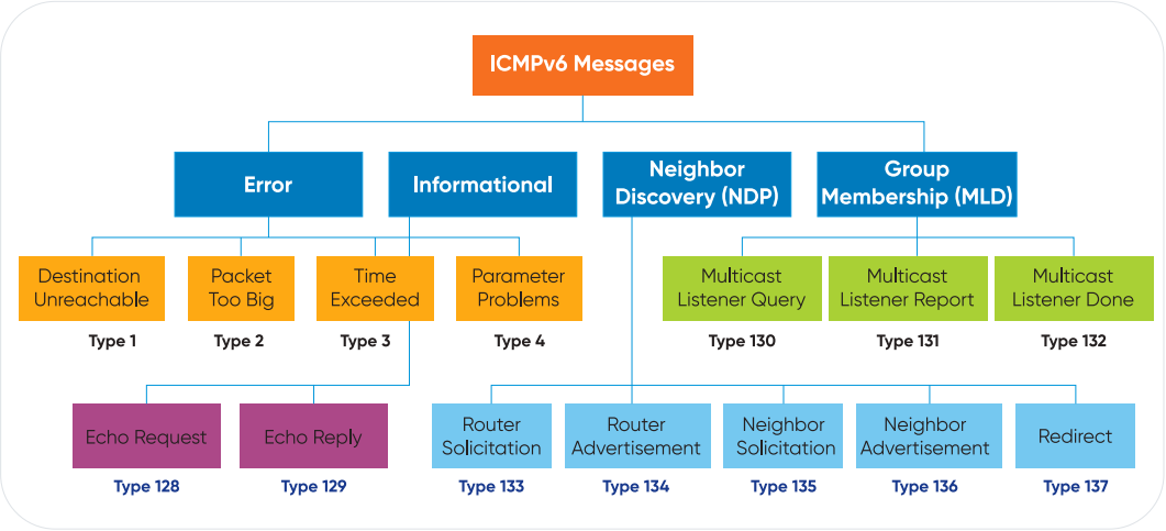
Hình 67. Chi tiết các bản tin của ICMPv6 và NDP, MLD
