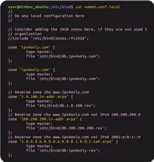
Hình 148. Khai báo cho named.conf.local
