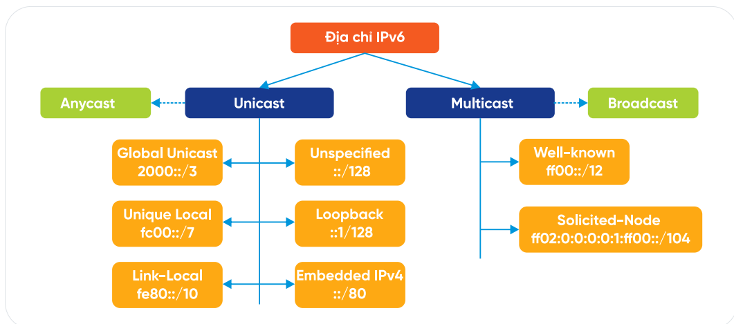
Hình 34. Chi tiết phân loại IPv6 theo cách thức và phạm vi hoạt động
