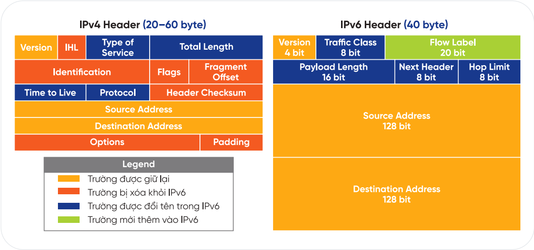
Hình 23. So sánh IPv4 và IPv6 Header
