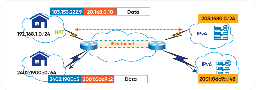
Hình 85. Hoạt động của cơ chế Tunnel
