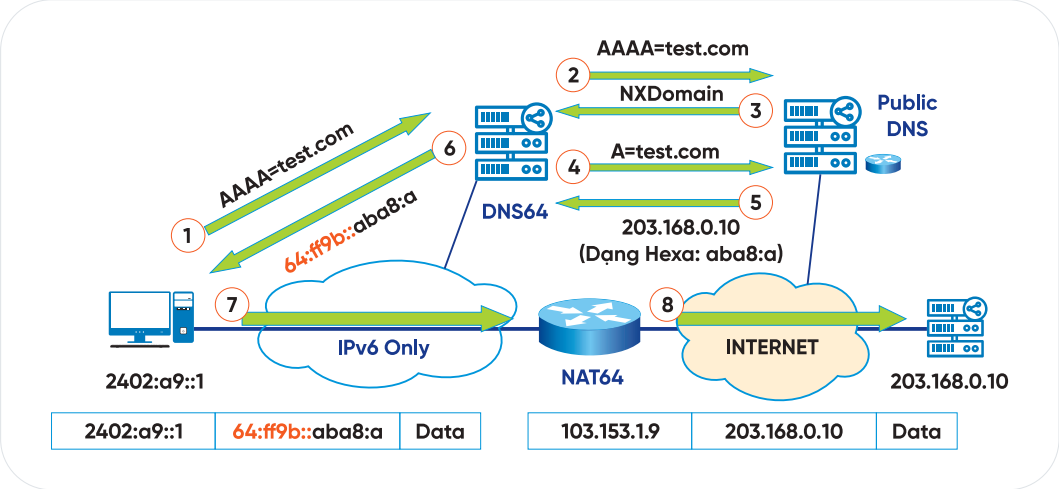
Hình 95. Nguyên tắc hoạt động của DNS64 và NAT64
