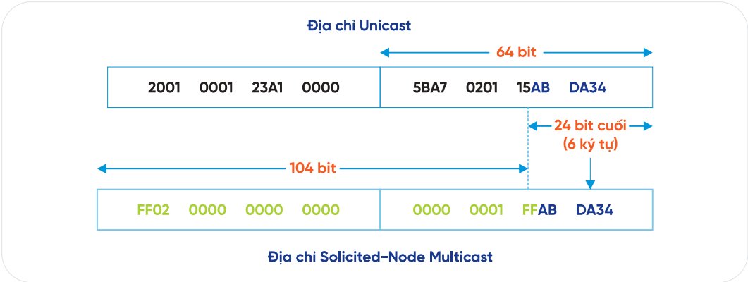
Hình 51. Ví dụ nguyên tắc tạo Solicited-Node Multicast từ Unicast
