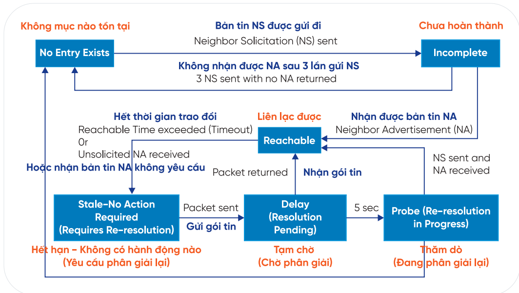
Hình 81. Chi tiết các trạng thái của Neighbor Cache
