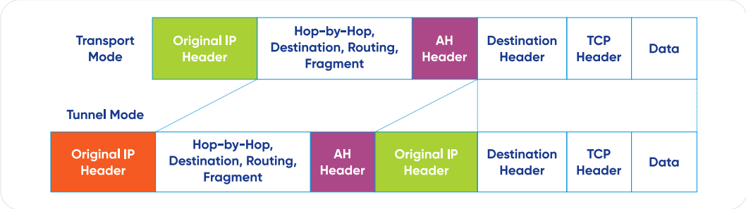
Hình 28. Vị trí AH và các Extension Header khác ở chế độ Transport và Tunnel
