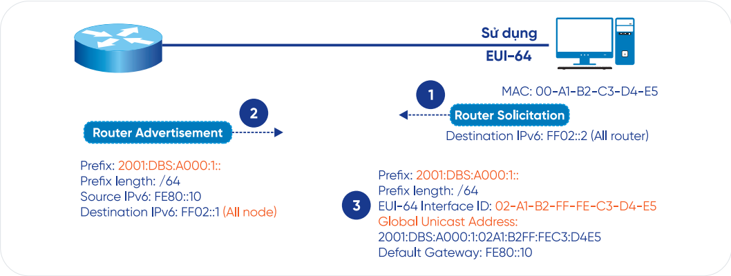
Hình 72. Chi tiết hoạt động của SLAAC
