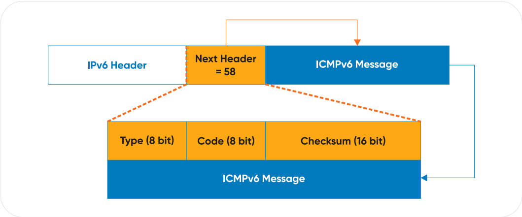
Hình 65. Định dạng chung của bản tin ICMPv6
