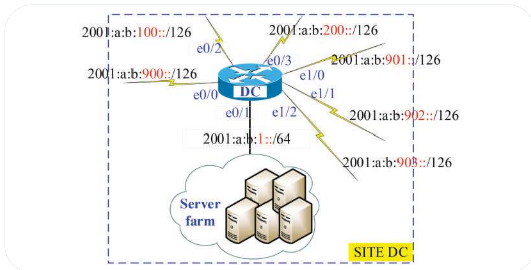
Hình 114. Chi tiết quy hoạch và phân bổ địa chỉ IPv6 cho các Level
