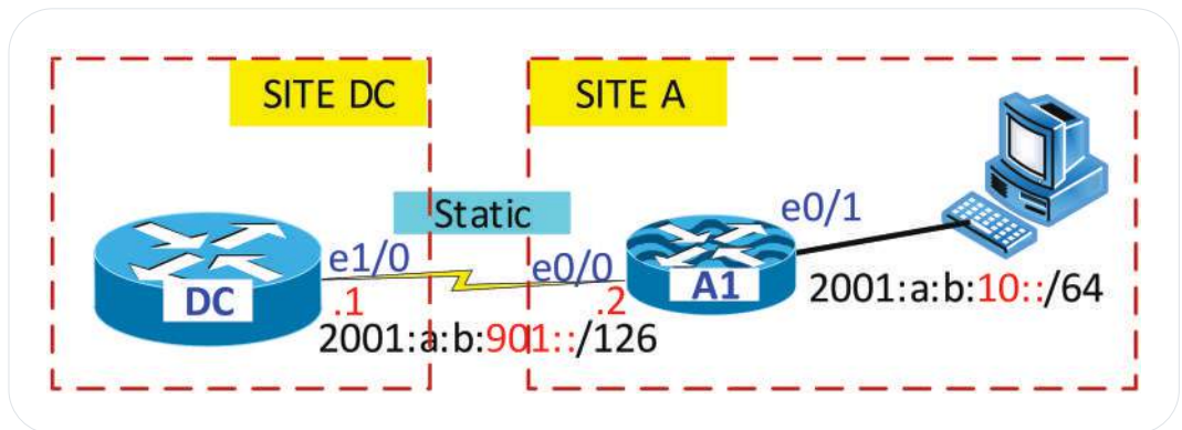
Hình 128. Mô hình của bài LAB về Static Route
