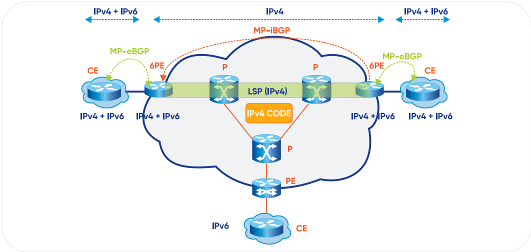
Hình 87. Hoạt động của cơ chế 6PE
