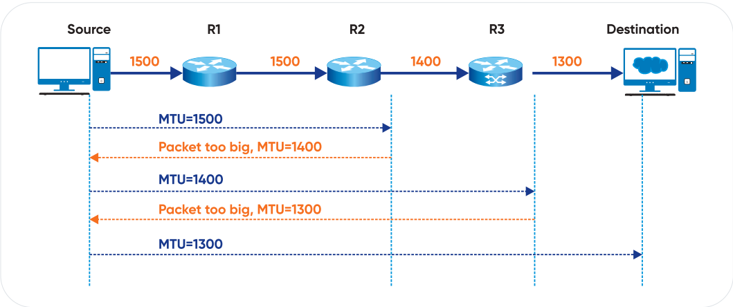
Hình 83. Hoạt động của IPv6 Path MTU
