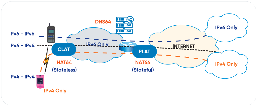
Hình 97. Nguyên tắc hoạt động của giải pháp DS-Lite
