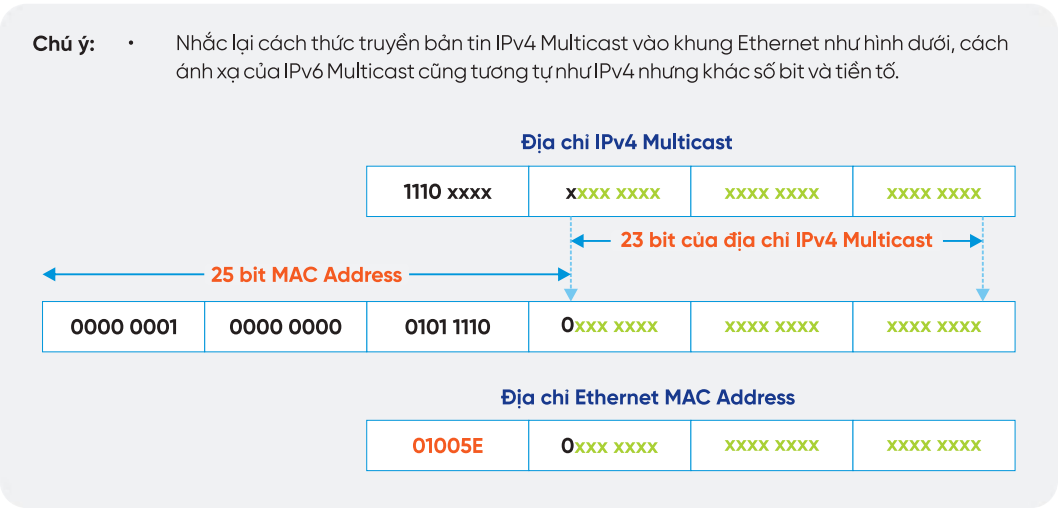
Hình 49. Ethernet Frame của bản tin IPv4 Multicast
