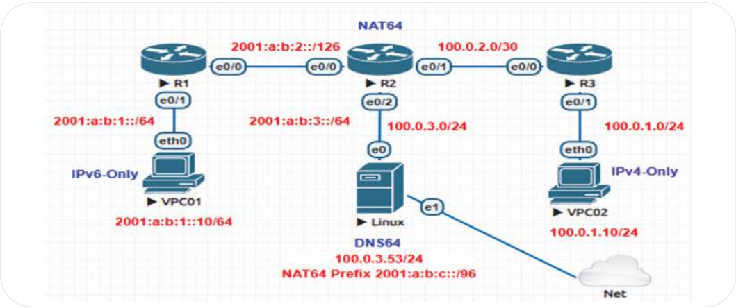
Hình 135. Mô hình LAB trên phần mềm EVE-NG
