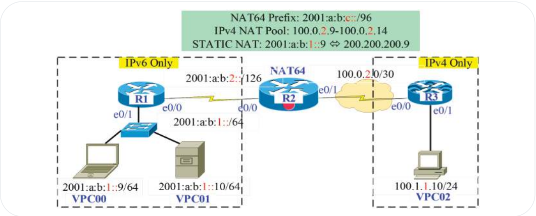
Hình 138. Mô hình của bài LAB về Static NAT64
