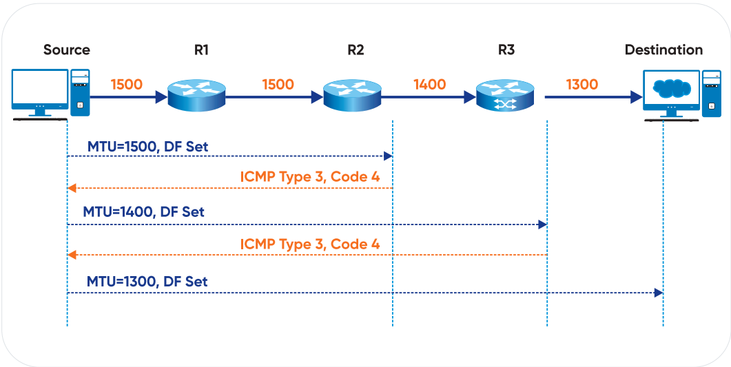
Hình 64. Chi tiết hoạt động của PMTU
