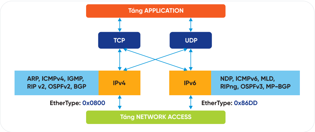
Hình 22. IPv4, IPv6 và các giao thức hỗ trợ
