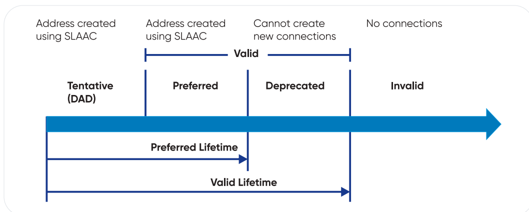
Hình 79. Các trạng thái của địa chỉ IPv6
