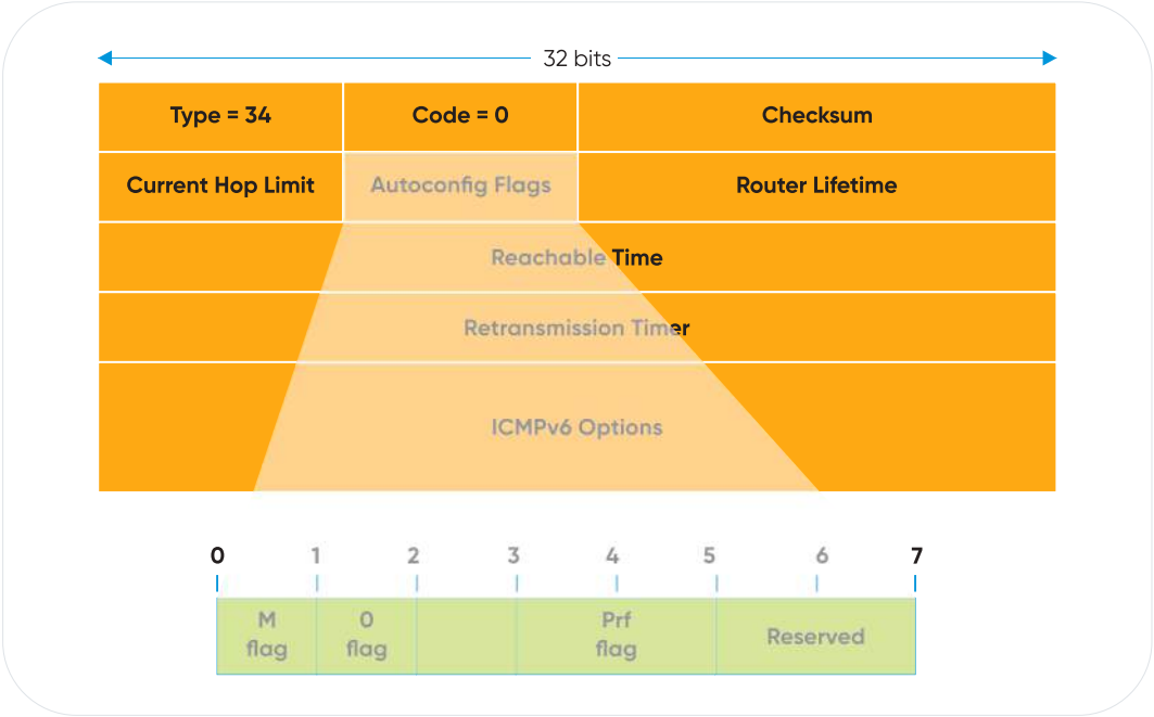
Hình 74. Cấu trúc bản tin Router Advertisement
