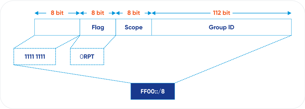
Hình 46. Cấu trúc của địa chỉ Multicast
