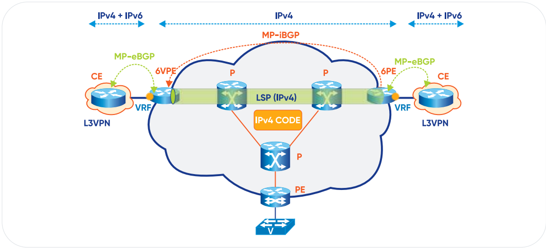
Hình 88. Hoạt động của cơ chế 6VPE
