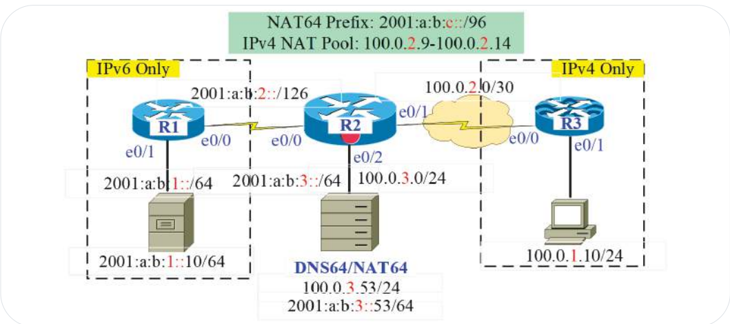
Hình 134. Mô hình LAB IPv6 Only với NAT64 và DNS64 được tích hợp
