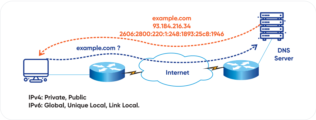
Hình 52. Minh họa truy cập Internet ở chế độ Dual Stack
