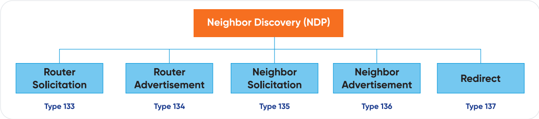
Hình 68. Chi tiết của các bản tin của NDP
