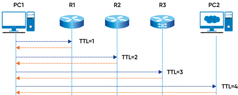
Hình 62. Chi tiết hoạt động của lệnh Trace
