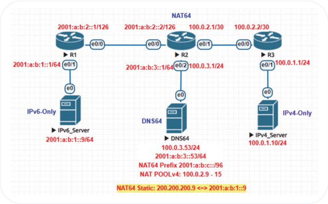
Hình 146. Mô hình của bài LAB sử dụng Dual Stack DNS64
