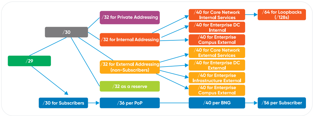
Hình 105. Ví dụ việc phân tầng cho nhà mạng
