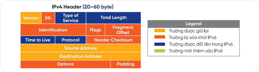
Hình 24. Những trường của IPv4 được giữ lại và bị xóa bỏ khỏi IPv6
