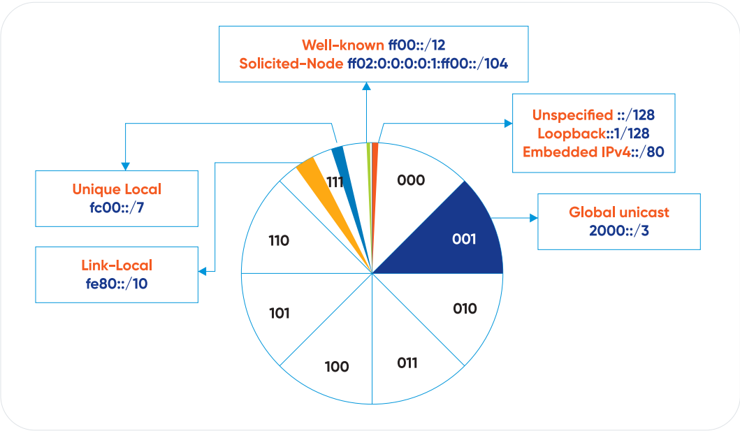
Hình 35. Chi tiết các loại địa chỉ IPv6 theo các phân vùng
