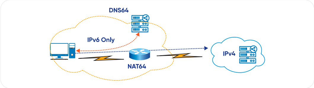
Hình 86. Kỹ thuật NAT cho mạng IPv6 Only
