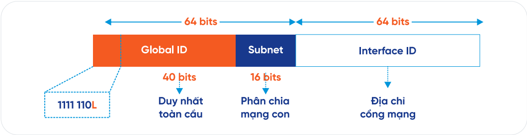
Hình 37. Cấu trúc của địa chỉ ULA
