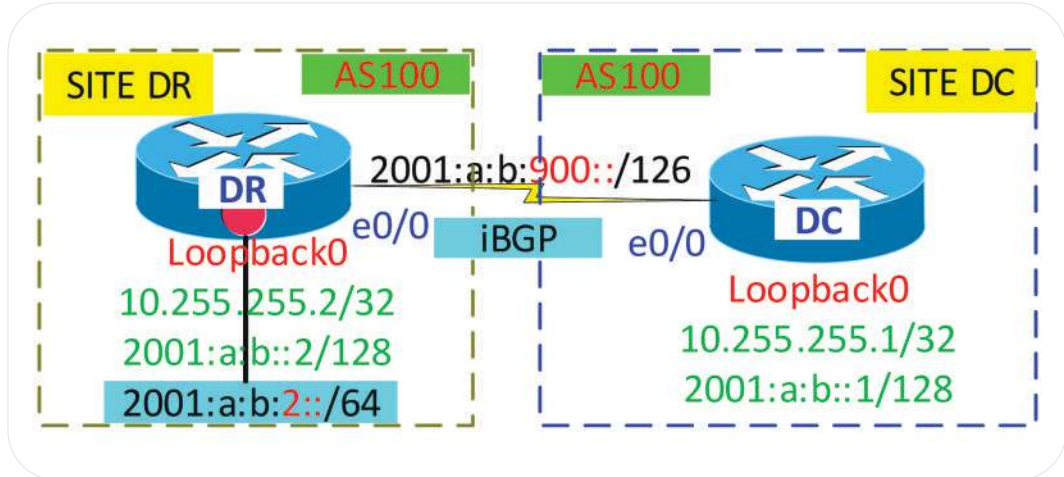
Hình 130. Mô hình của bài LAB về iBGP
