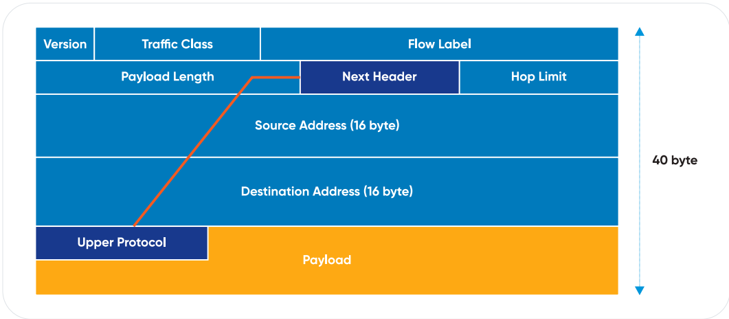
Hình 26. Ý nghĩa của trường Next Header
