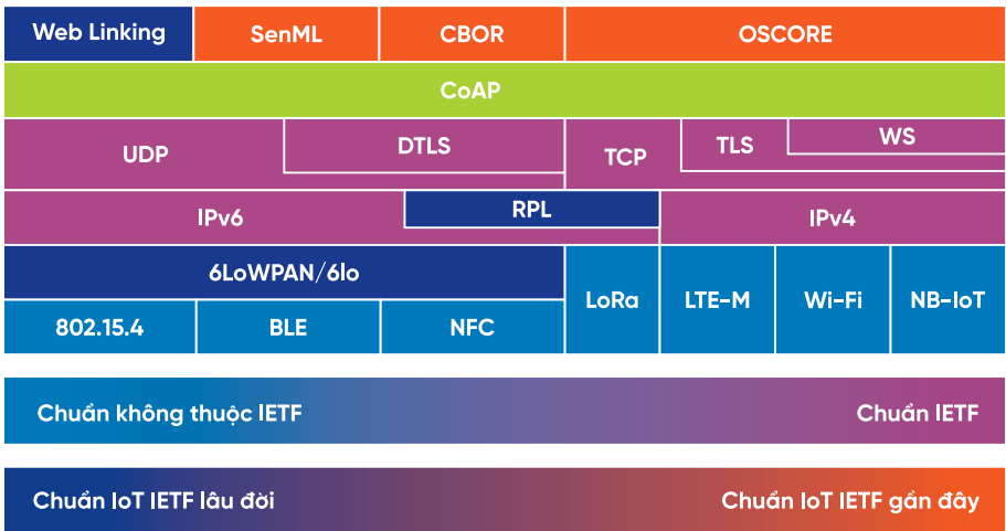
Hình 15. Các chuẩn giao thức IoT liên quan đến IPv6
