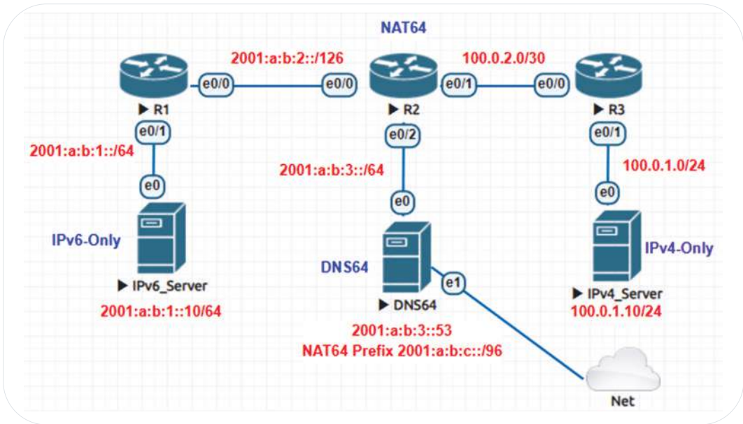
Hình 139. Mô hình của bài LAB sử dụng IPv6 Only DNS64
