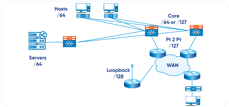
Hình 102. Một số Prefix Length đặc biệt
