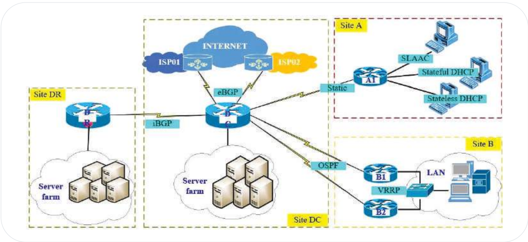
Hình 112. Mô hình LAB tổng thể
