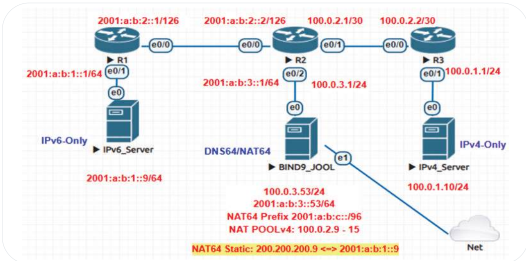
Hình 157. Mô hình của bài LAB IPv6 Only tích hợp giữa NAT64 và DNS64
