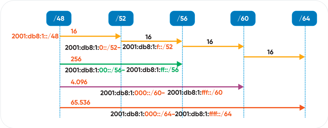
Hình 99. Cách thức phân chia theo Nibble
