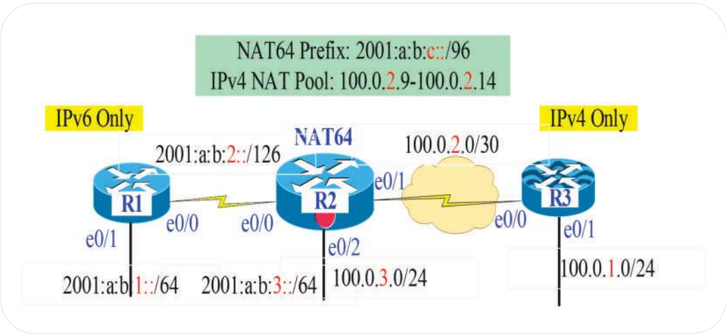
Hình 136. Mô hình của bài LAB về Dynamic NAT64
