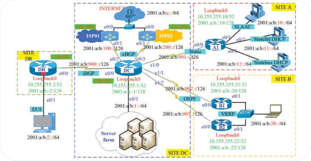
Hình 113. Chi tiết thông tin quy hoạch cho bài LAB
