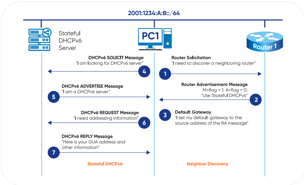
Hình 76. Chi tiết hoạt động của Stateful DHCPv6
