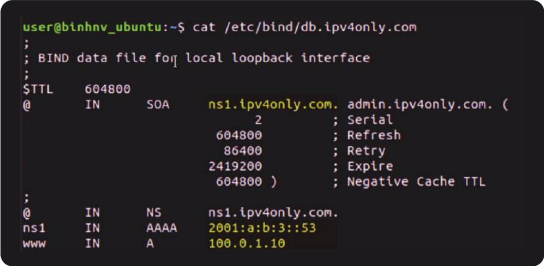
Hình 142. Khai báo cho db.ipv4only.com
