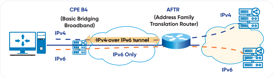
Hình 96. Nguyên tắc hoạt động của giải pháp DS-Lite
