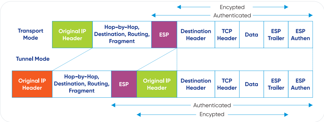
Hình 29. Vị trí ESP và các Extension Header khác ở chế độ Transport và Tunnel
