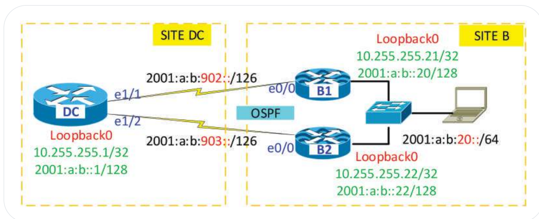
Hình 129. Mô hình của bài LAB về OSPFv3
