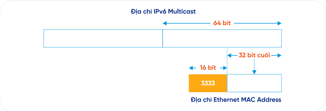
Hình 48. Ethernet Frame của bản tin IPv6 Multicast
