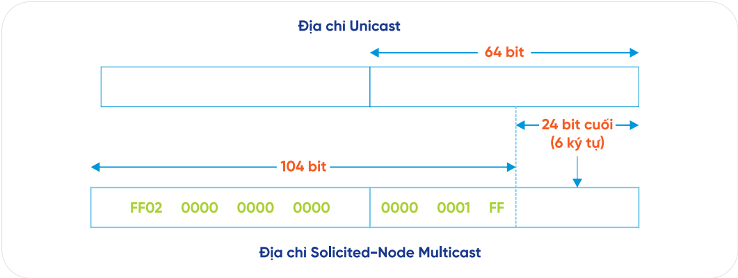
Hình 50. Nguyên tắc tạo Solicited-Node Multicast từ Unicast
