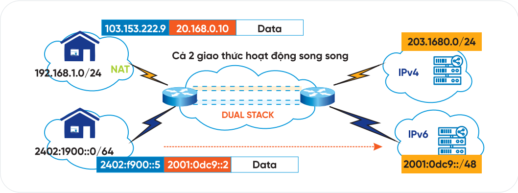
Hình 84. Hoạt động của cơ chế Dual Stack
